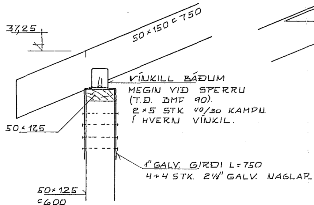
SERMYND B 1:10
