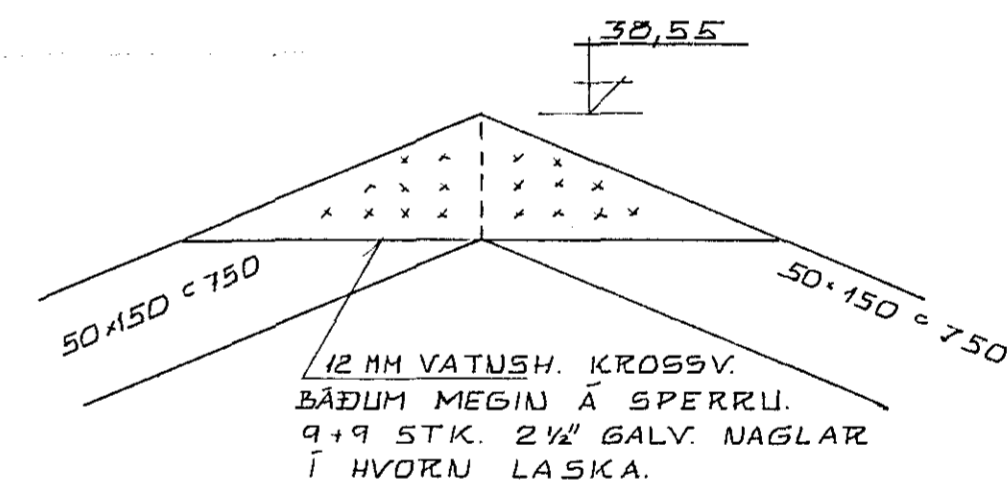
SERMYND D 1:10
