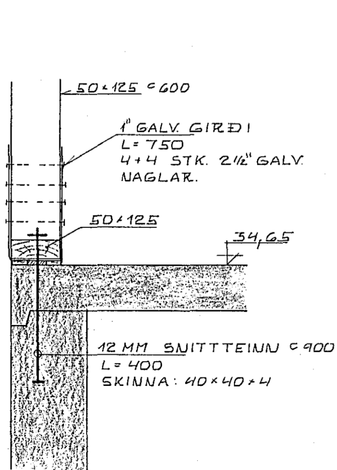
SERMYND A 1:10
