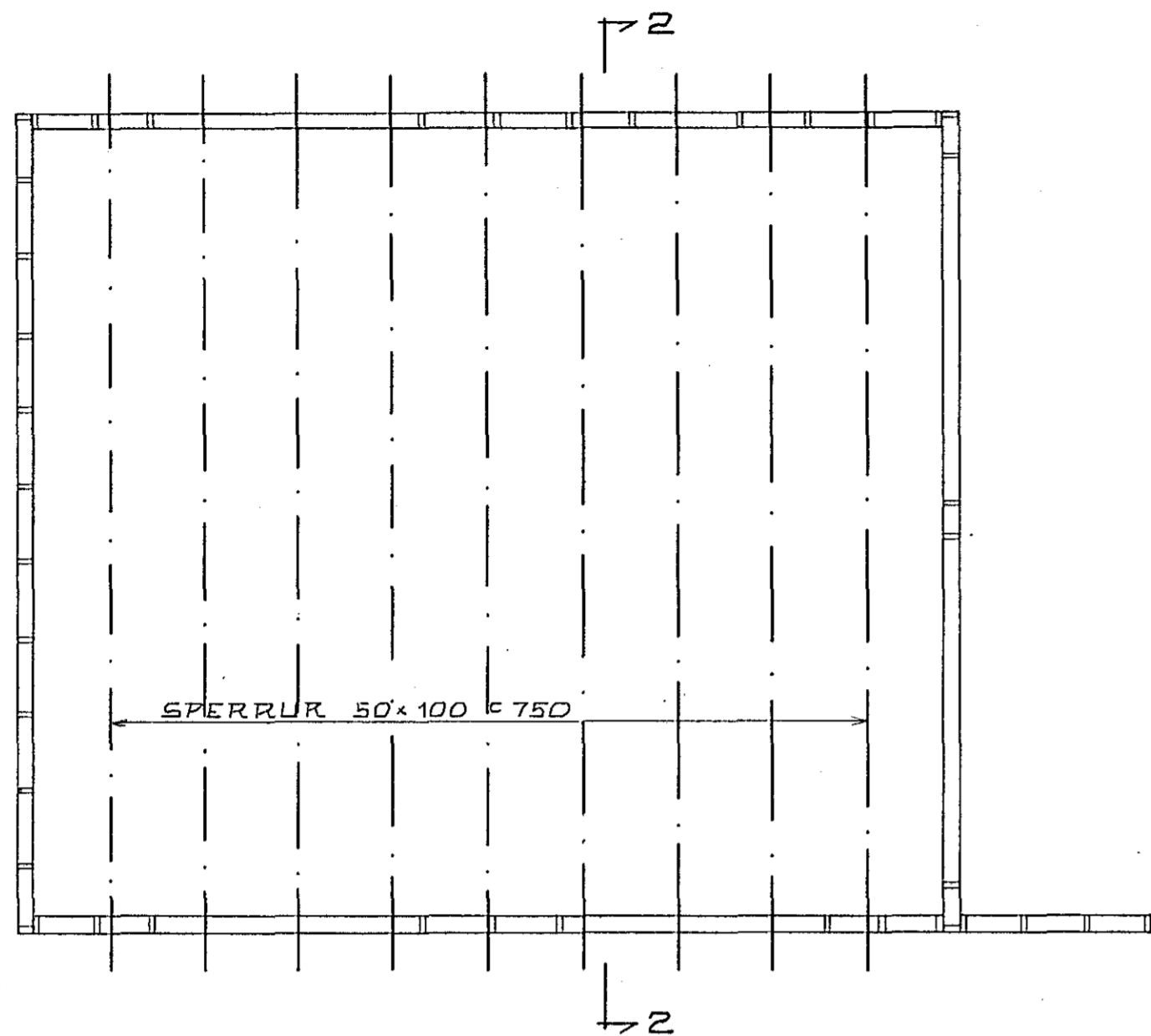
GRUNNMYND 1:50
