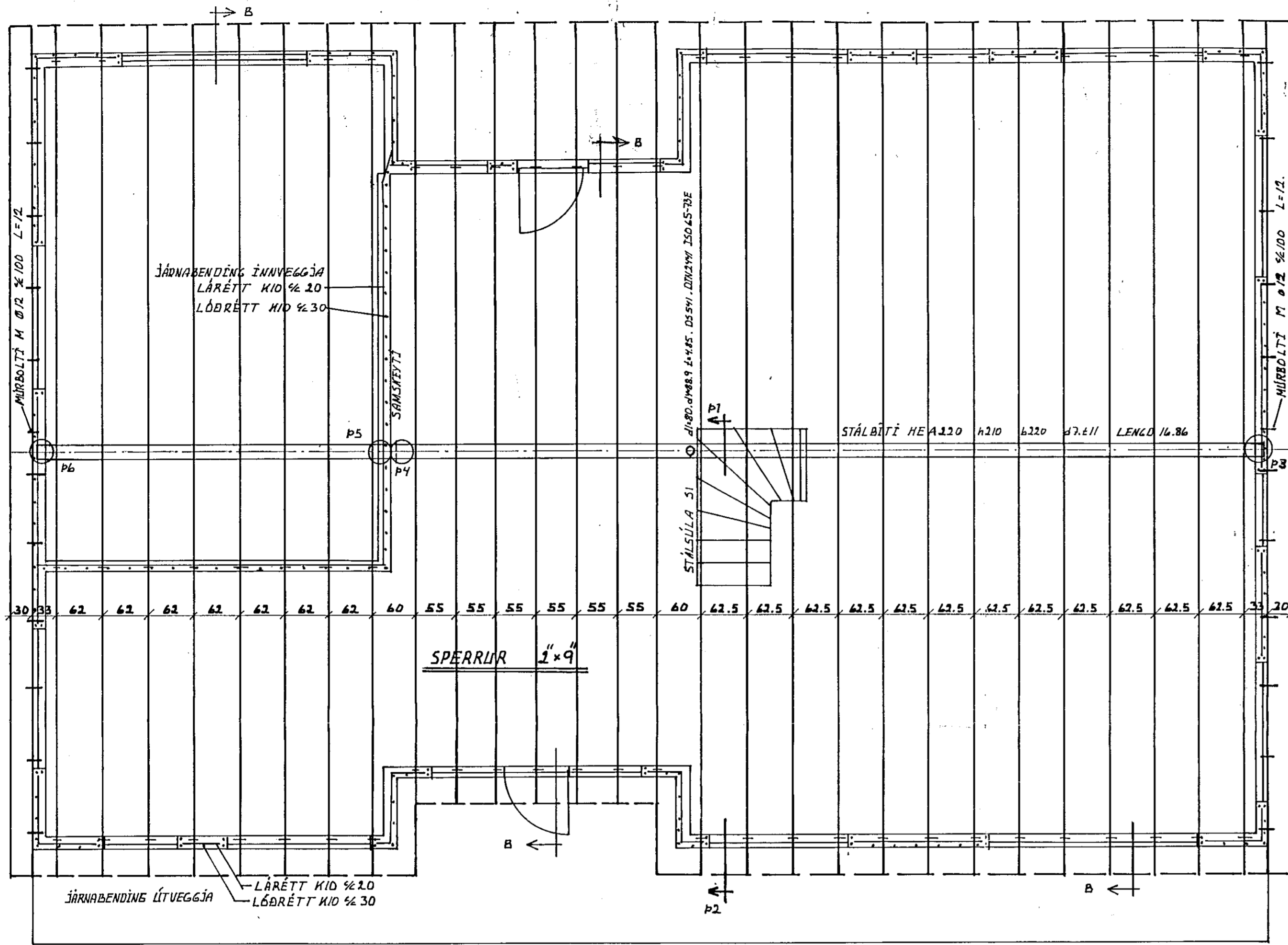
JÄRNABENDING VEGGJA. GRUNNMYND ÞAKVIRKIS. Mkv.: 1:50
