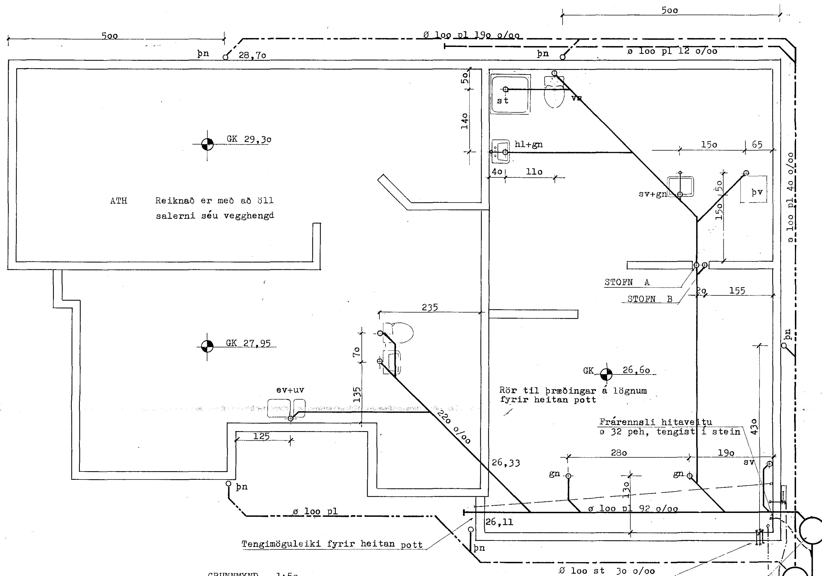
GRUNNMYND 1:50
