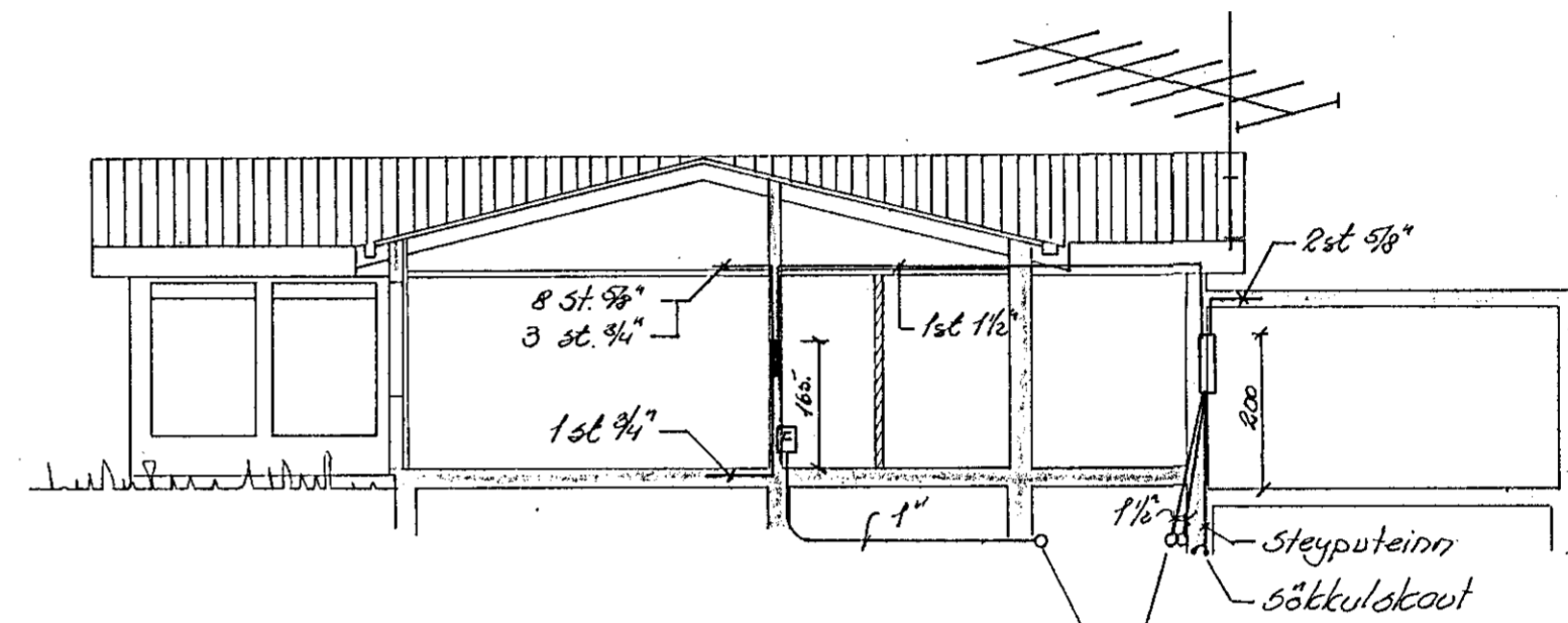
Sníð A-A 1:100
