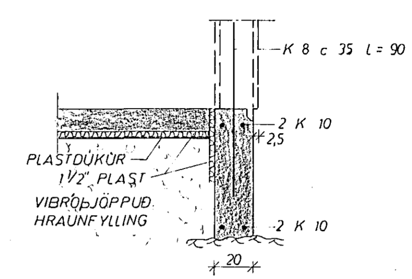
SNID 'I' ÚTVEGG 1:20
