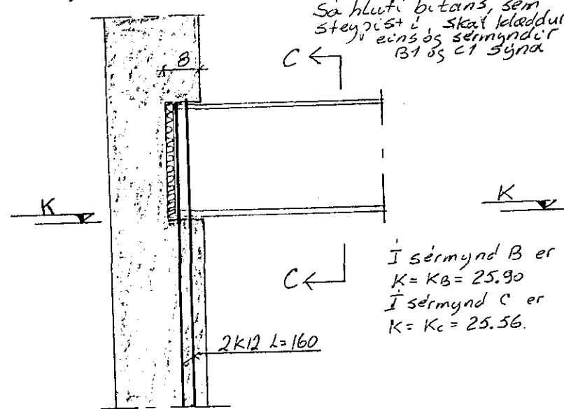
Sérmyndir B og C M. 1:10
