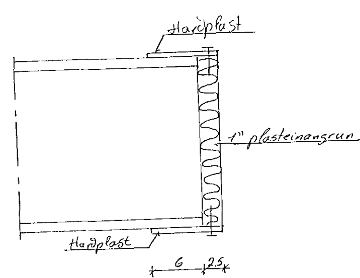
Snið D-D M. 1:5
