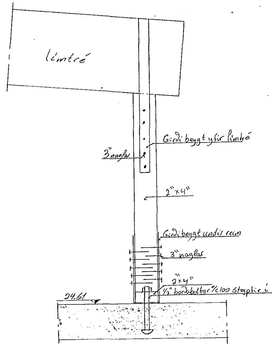
Sérmynd D M. 1:10
