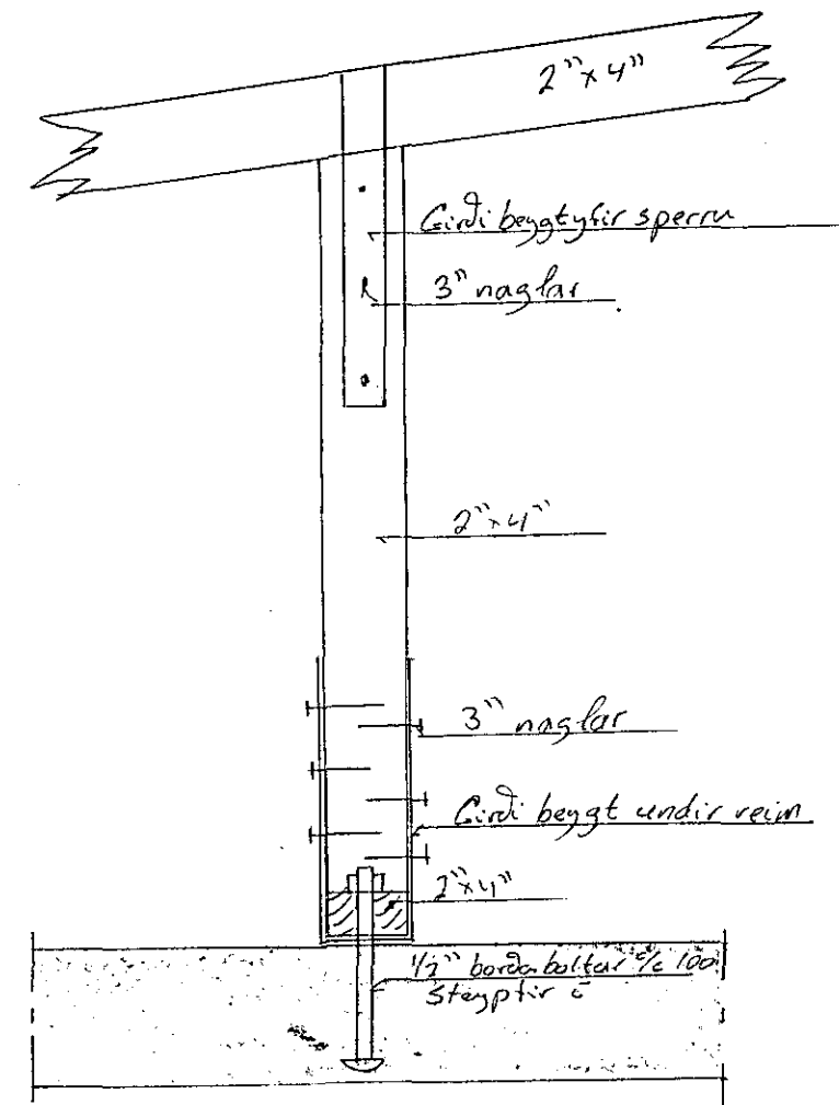
Sérmynd af stöla- og reima festingum M. 1:10
