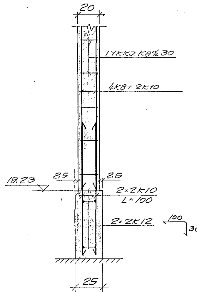
SNID E-E. 1:20 SÜLA S1
