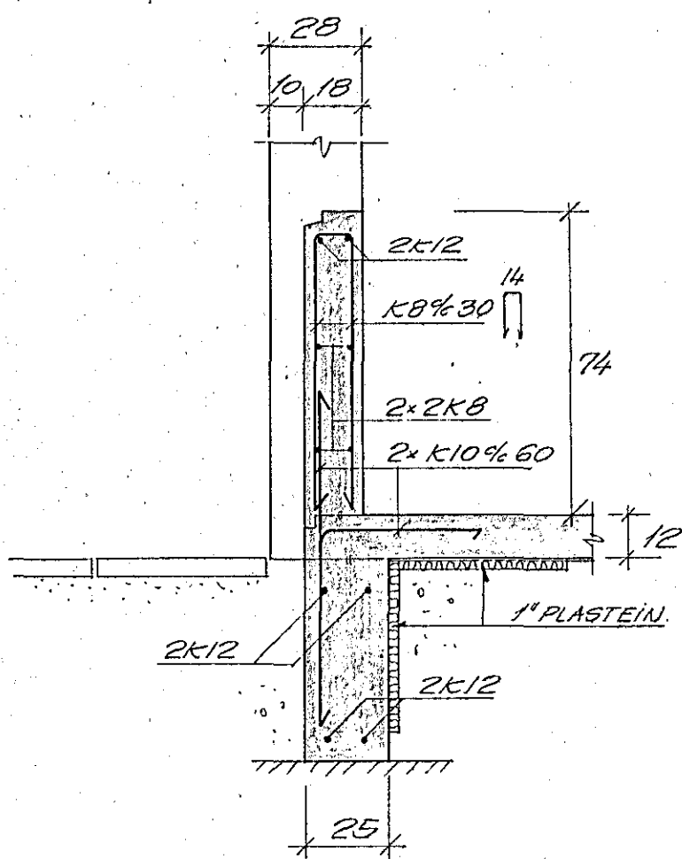
SNID D-D. 1:20 BENDING I SÖLU EKKI SYND
