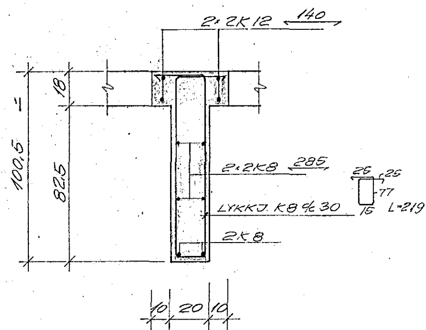
SÜLA S3. 1:20
