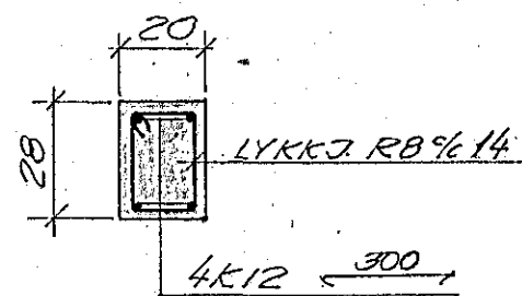
SÜLA S3. 1:20
