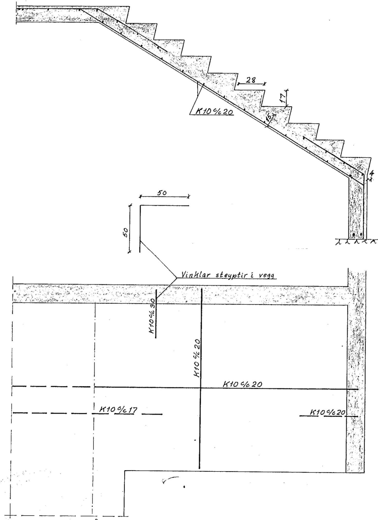
SNID I STIGA FRÁ SVÖLLUM M 1:20
