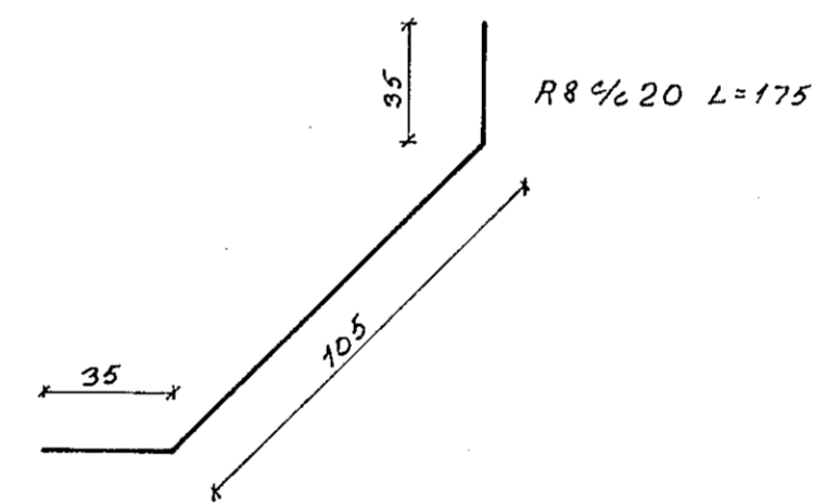
SNID I REYKHÁF M 1:20
