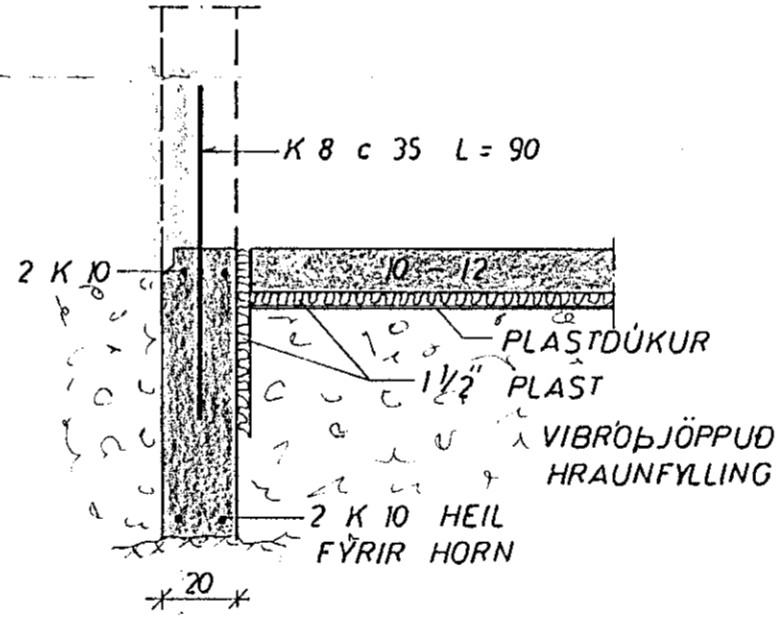
SNID '1 ÚTVEGG 1:20
