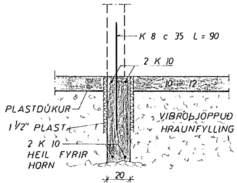
SNID '1 INNVEGG 1:20
