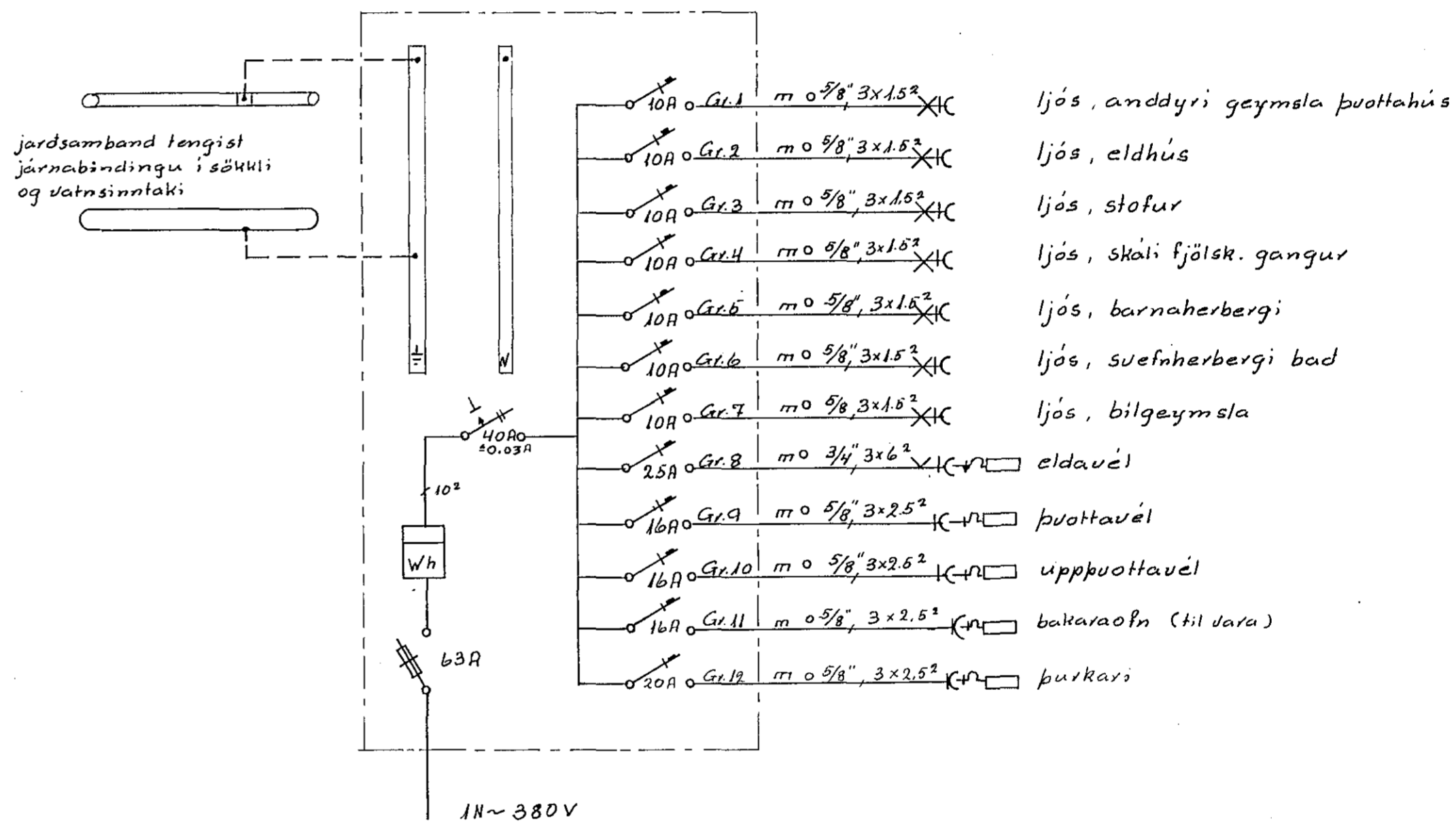
Einlinumynd
