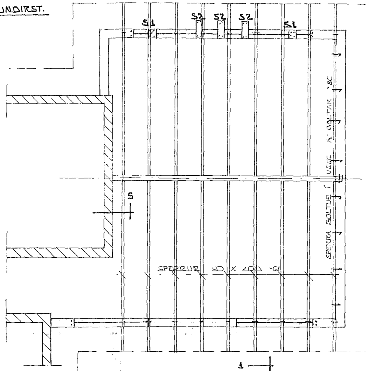
GRUNNMYND BURÐARVIRKI ~ 1:50
