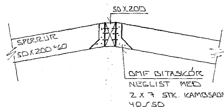
SERMYND 3 ~ 1:20
