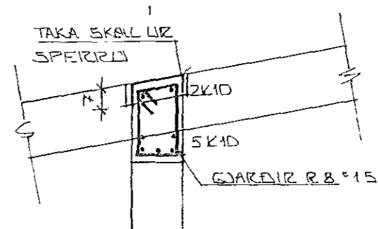
SERMYND 2 ~ 1:20
