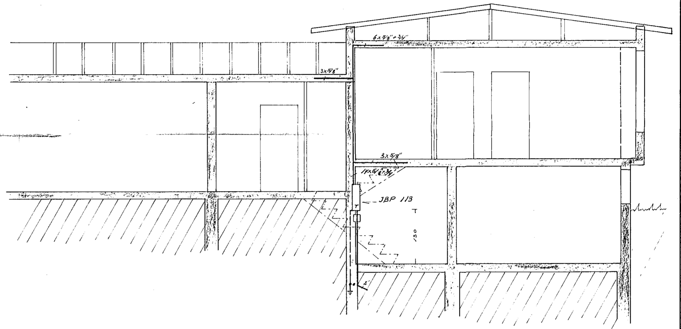
snid A-A
