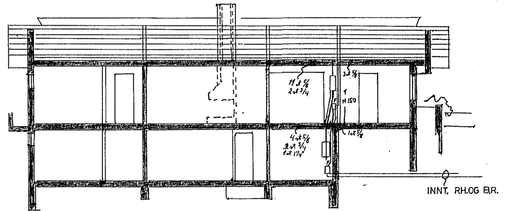
SKURÐUR M 1:100
