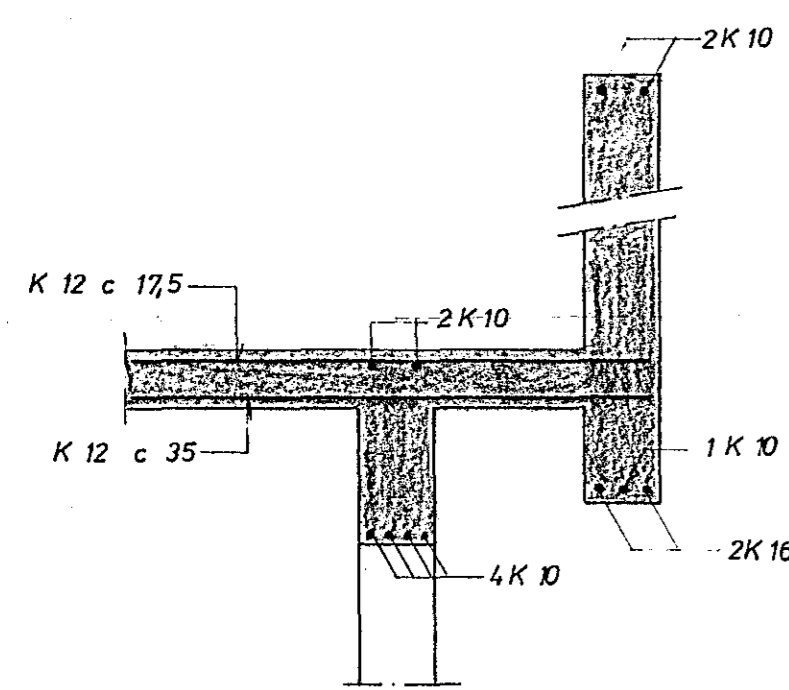
SNID E 1:20
