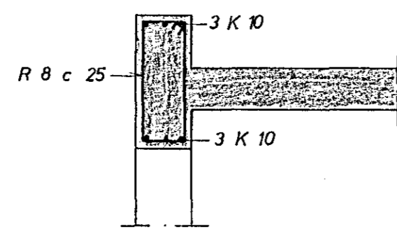
SNID D 1:20
