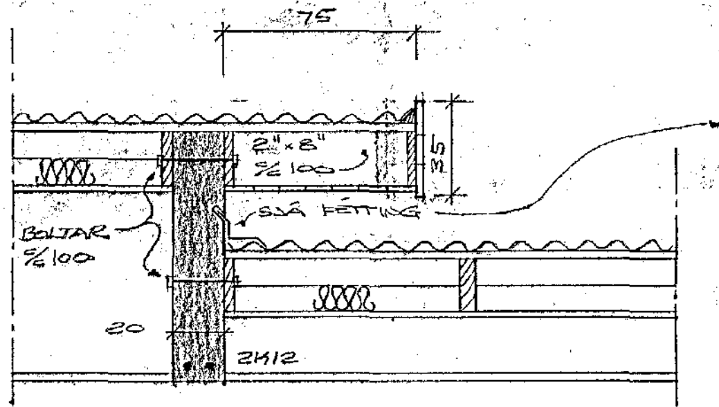
SKURDUR F. M=1:20
