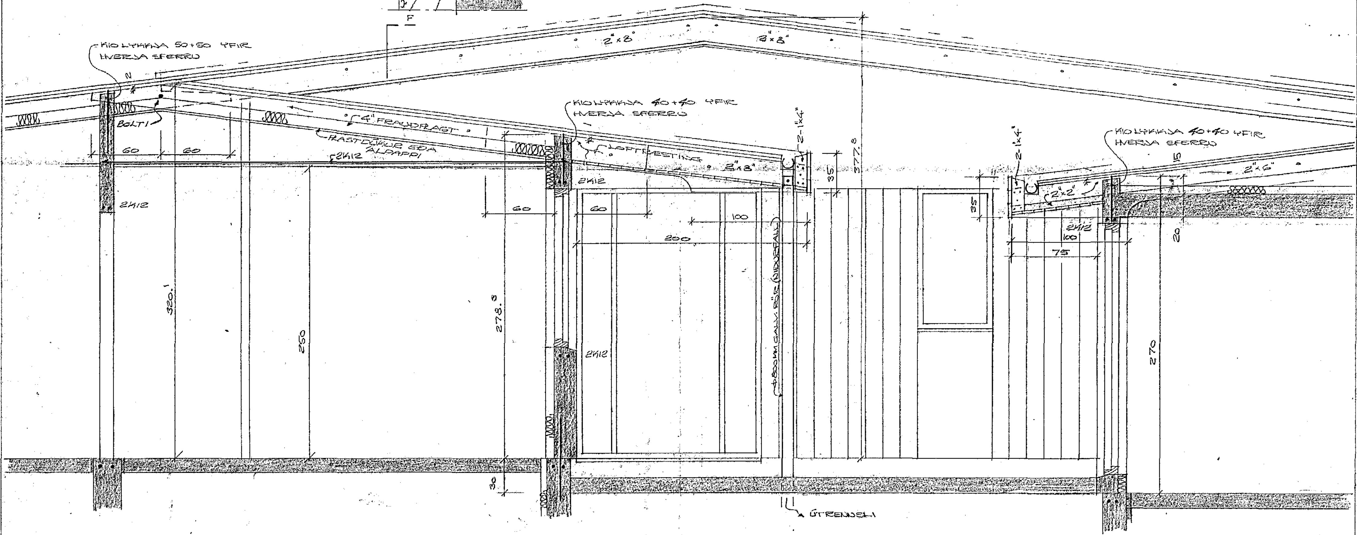
SKURDUR D. M=1:20
