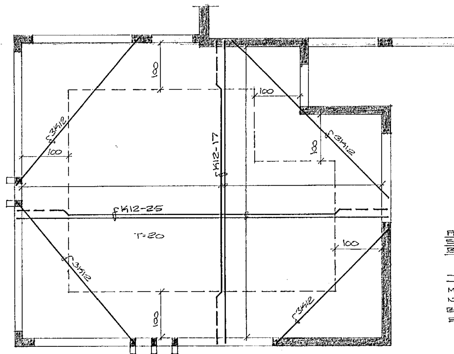
GRUNNMYND. M=1:50
