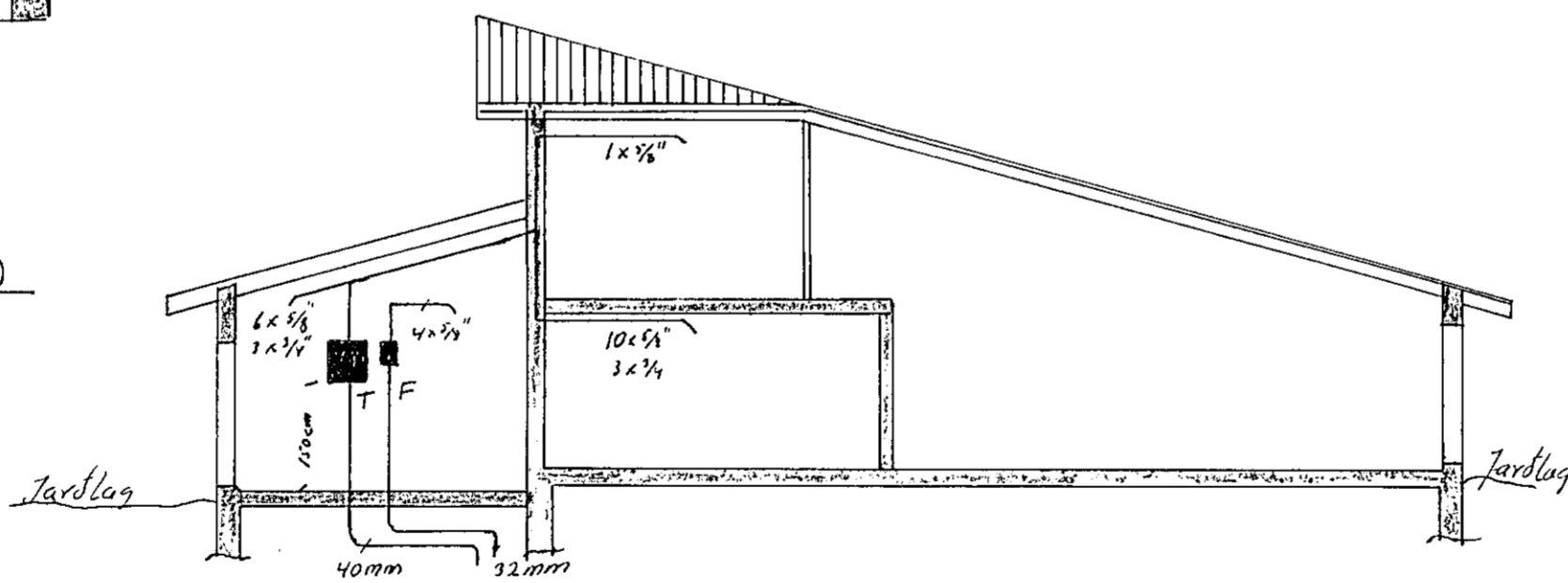
Snið. 1:100
