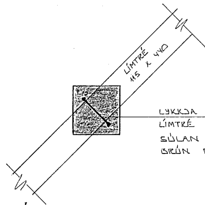
DEILI A ~ 1:10 TEIKN 10
