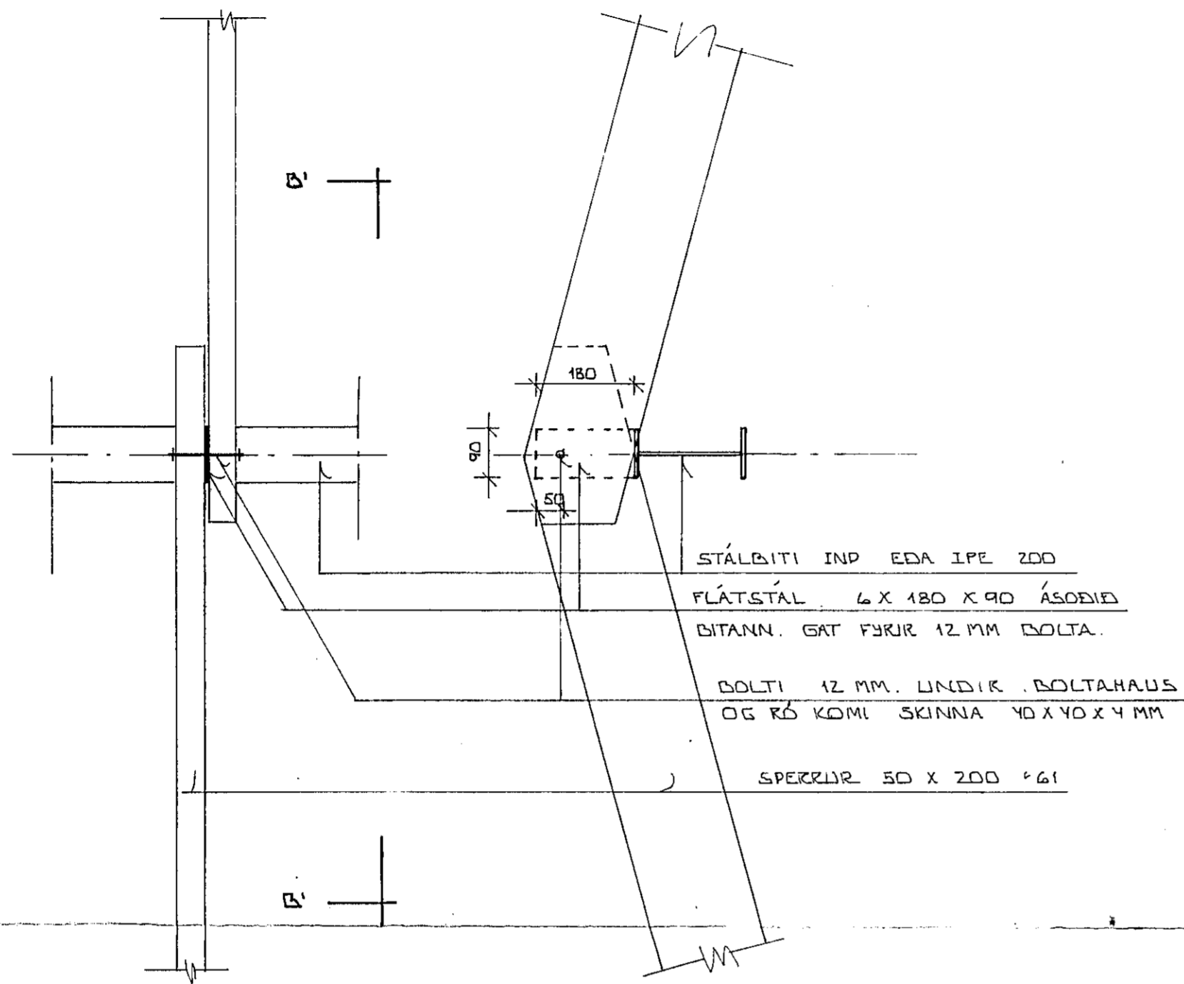
SNID B' - B' ~ 1:10
