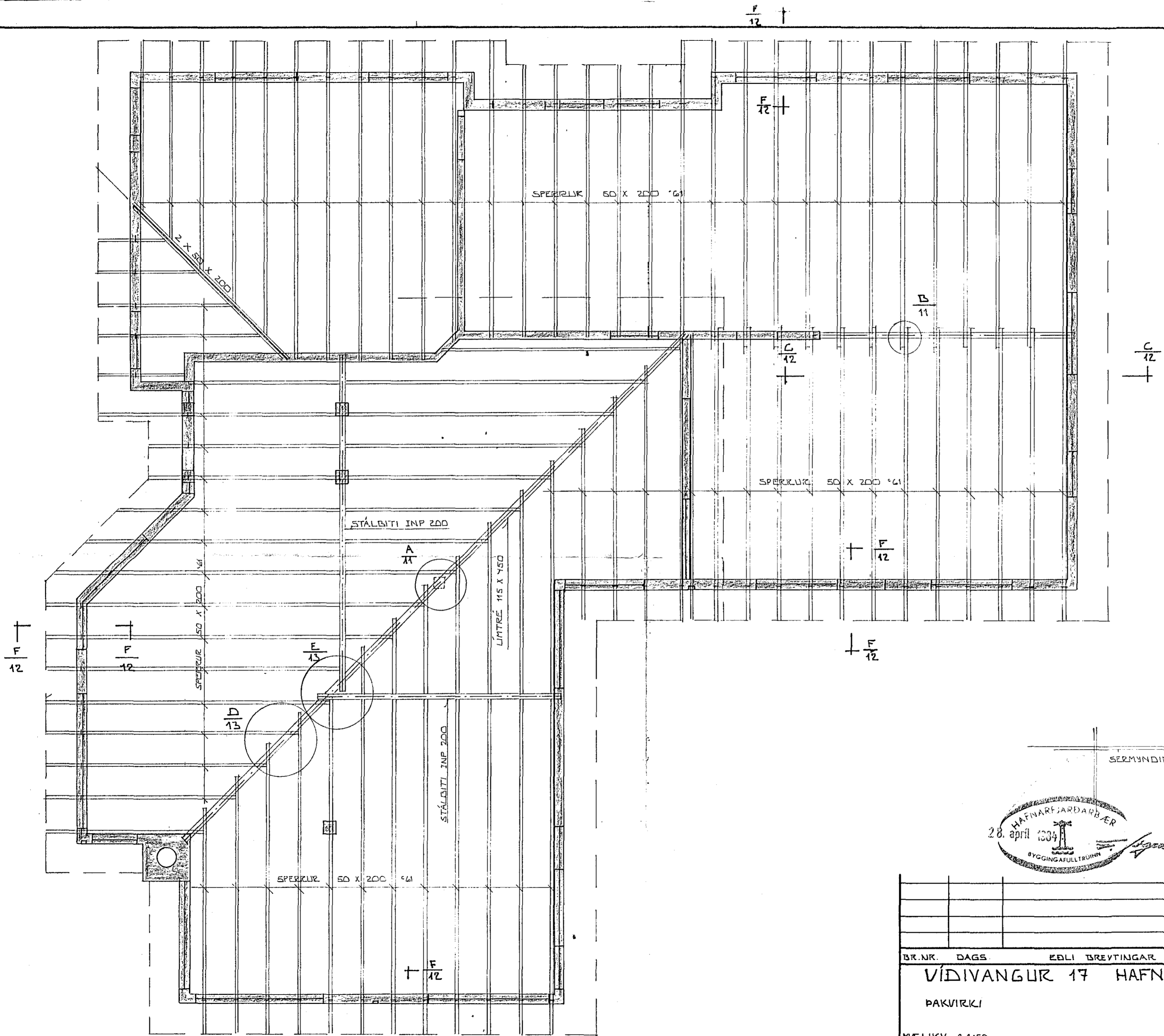
GRUNNMYND ~ 1:50
