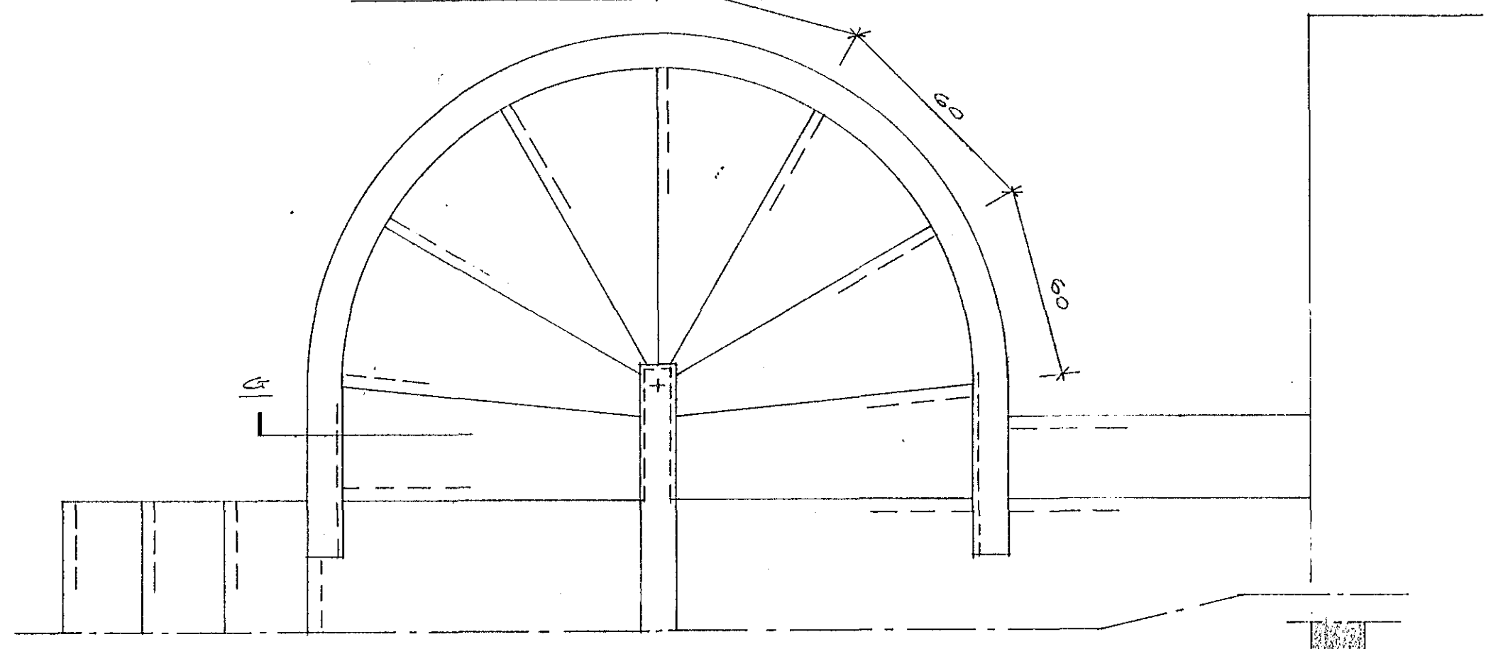
GRUNNMÓND. M. 1:20
