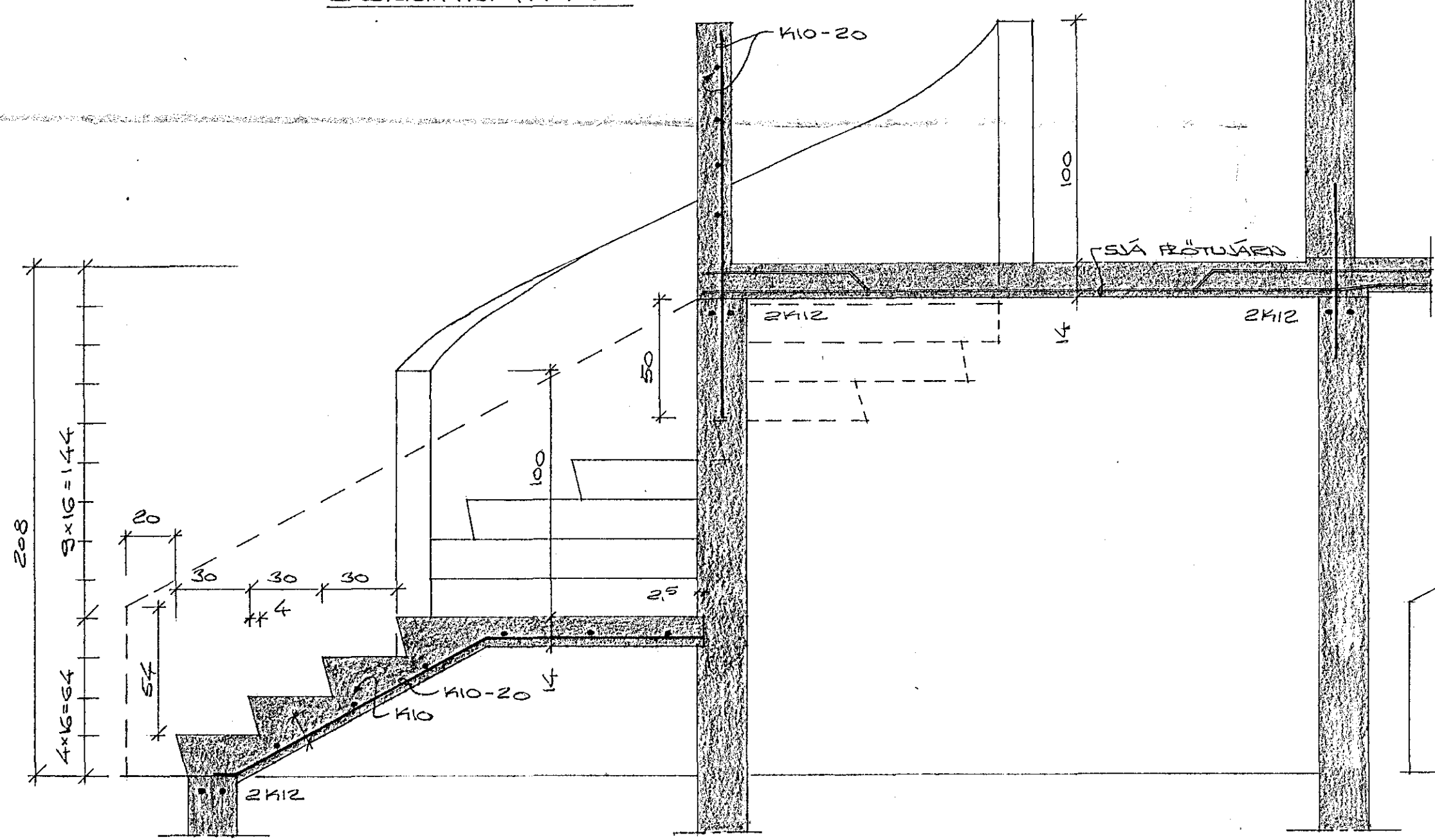
SKURÐUR E. M. 1:20
