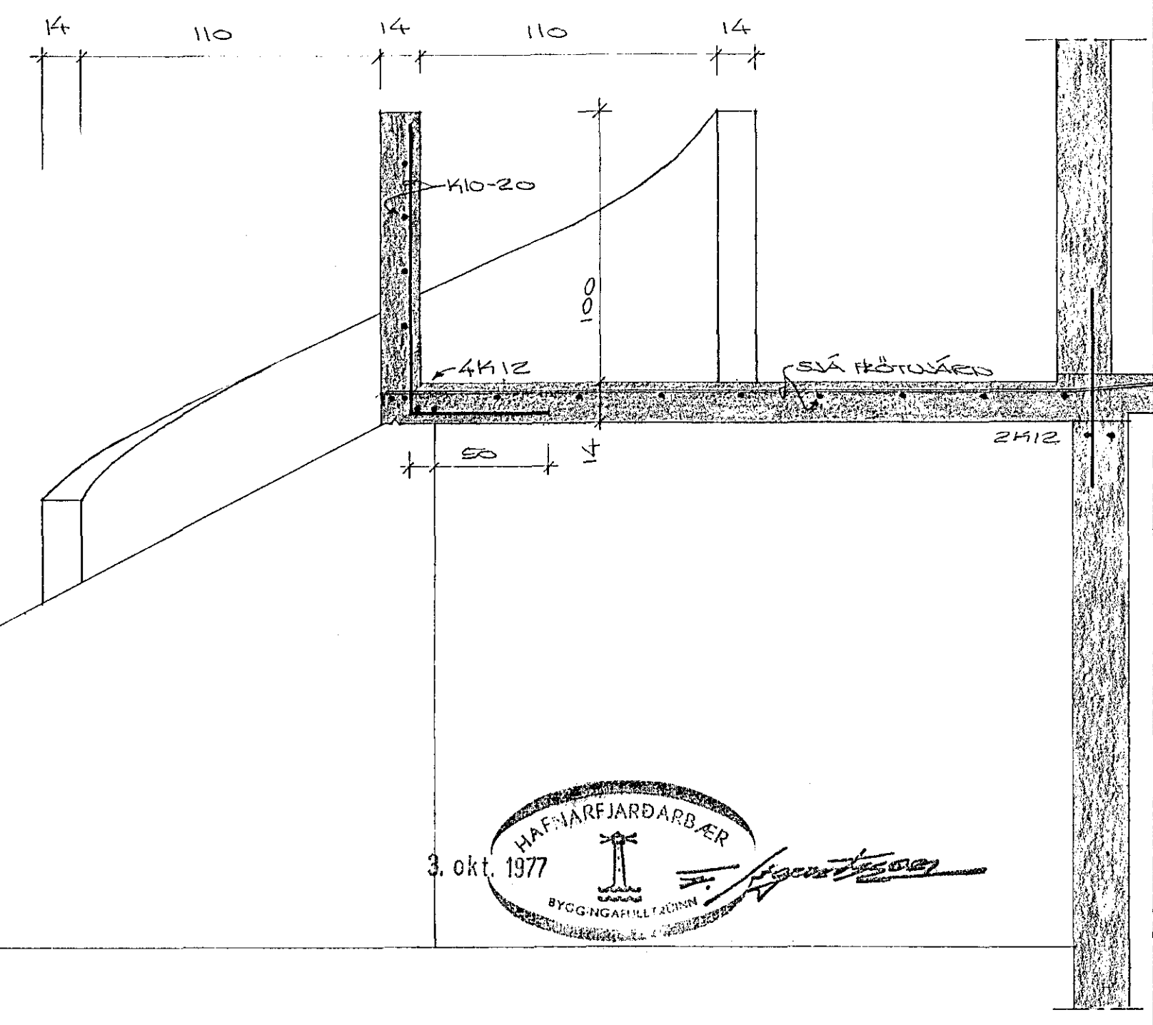
SKURÐUR F. M. 1:20
