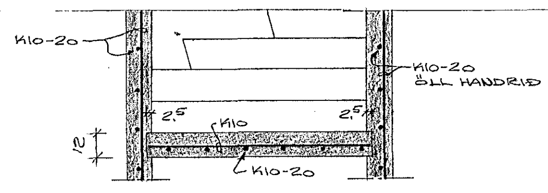
SKURÐUR G. M. 1:20
