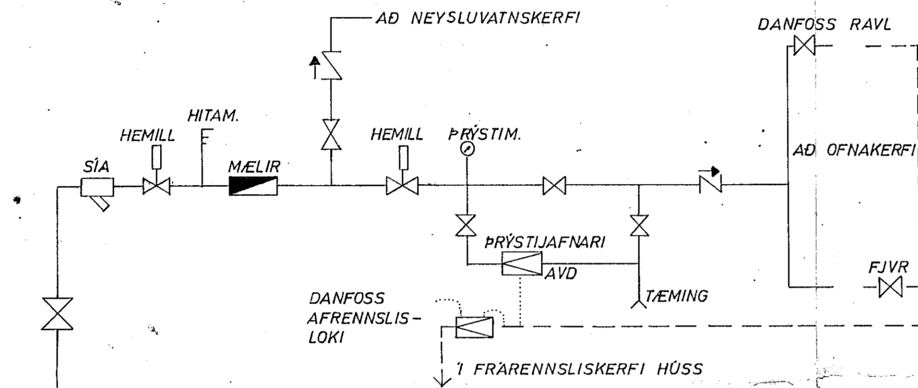
TENGIMYND HITAVEITU
