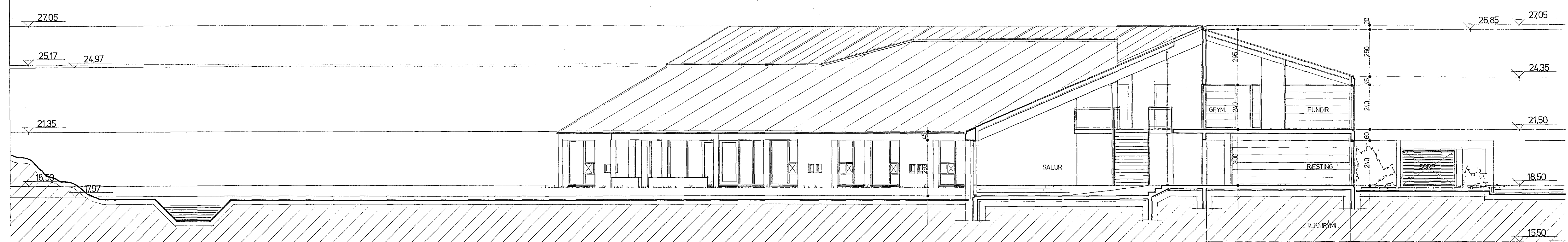
SNEIÐING B-B
