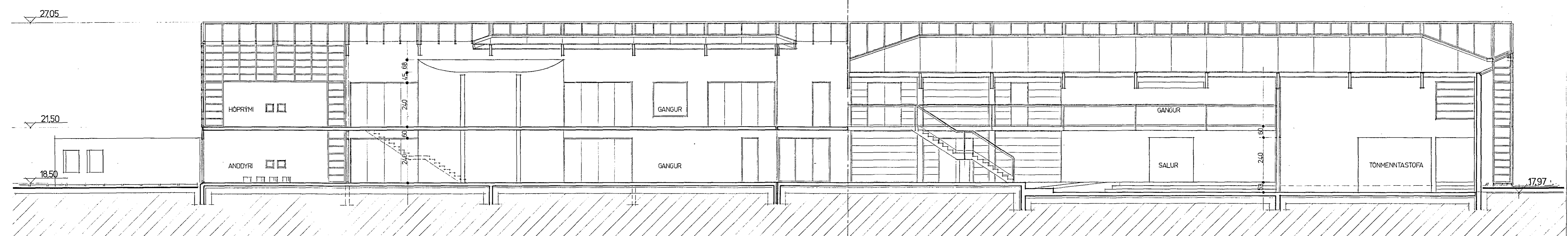
SNEIÐING C-C
