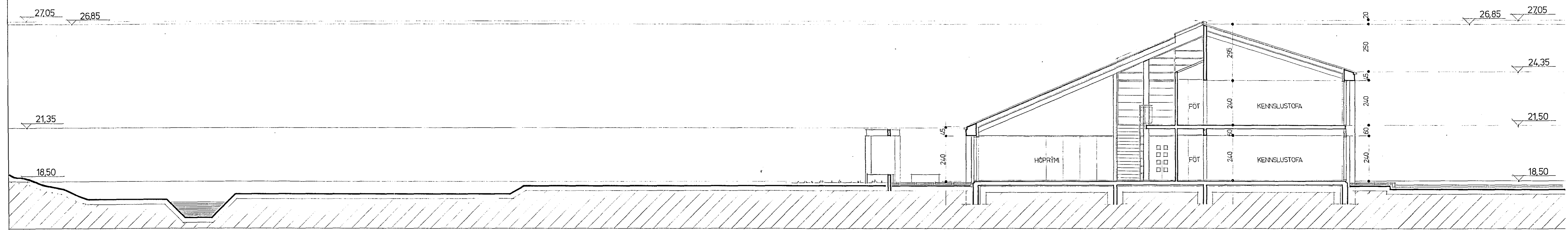
SNEIÐING A-A
