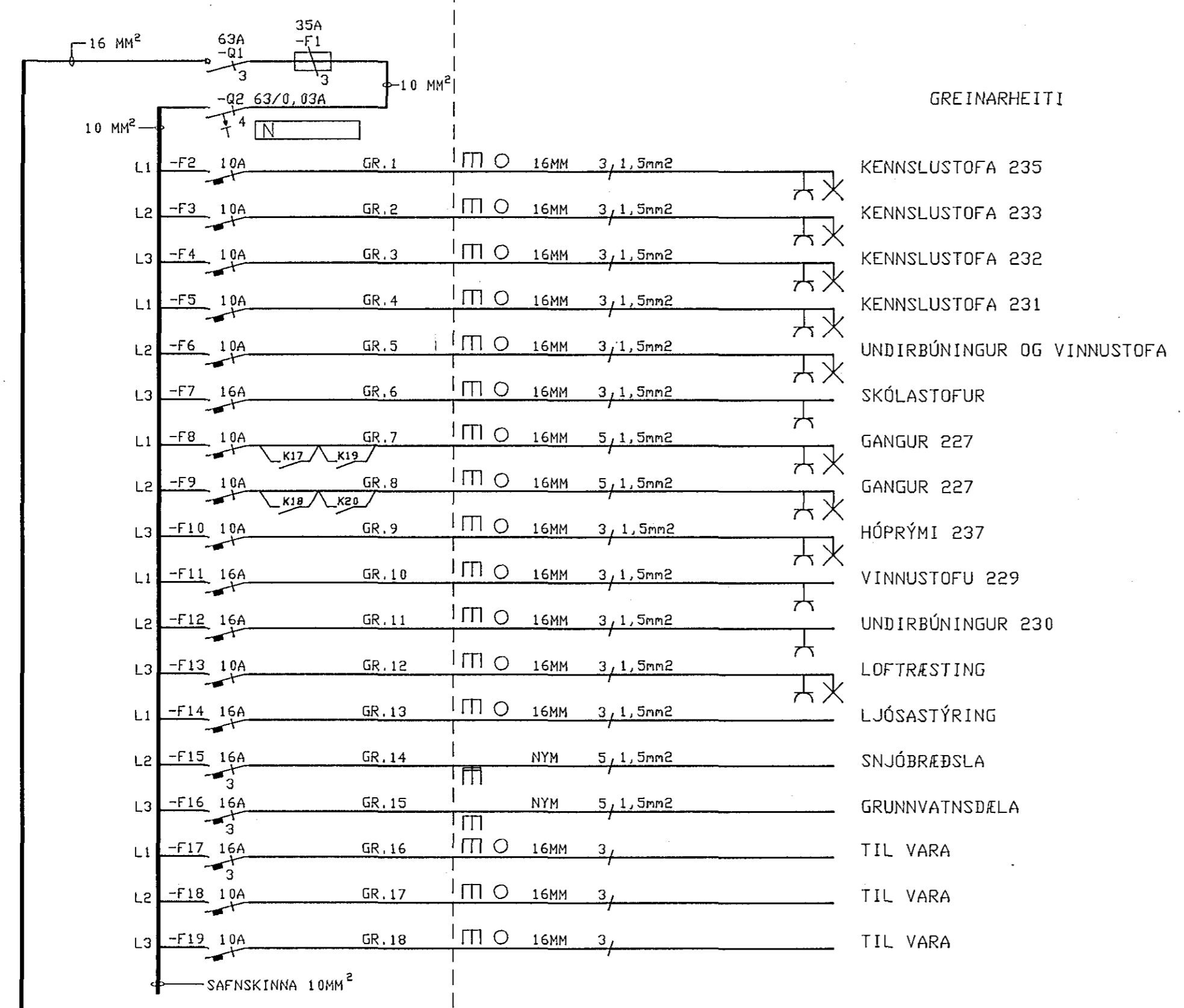
TAFLA T1.6 LÖFTRÆSTIKLEFA 3N 380 V 50 Hz
