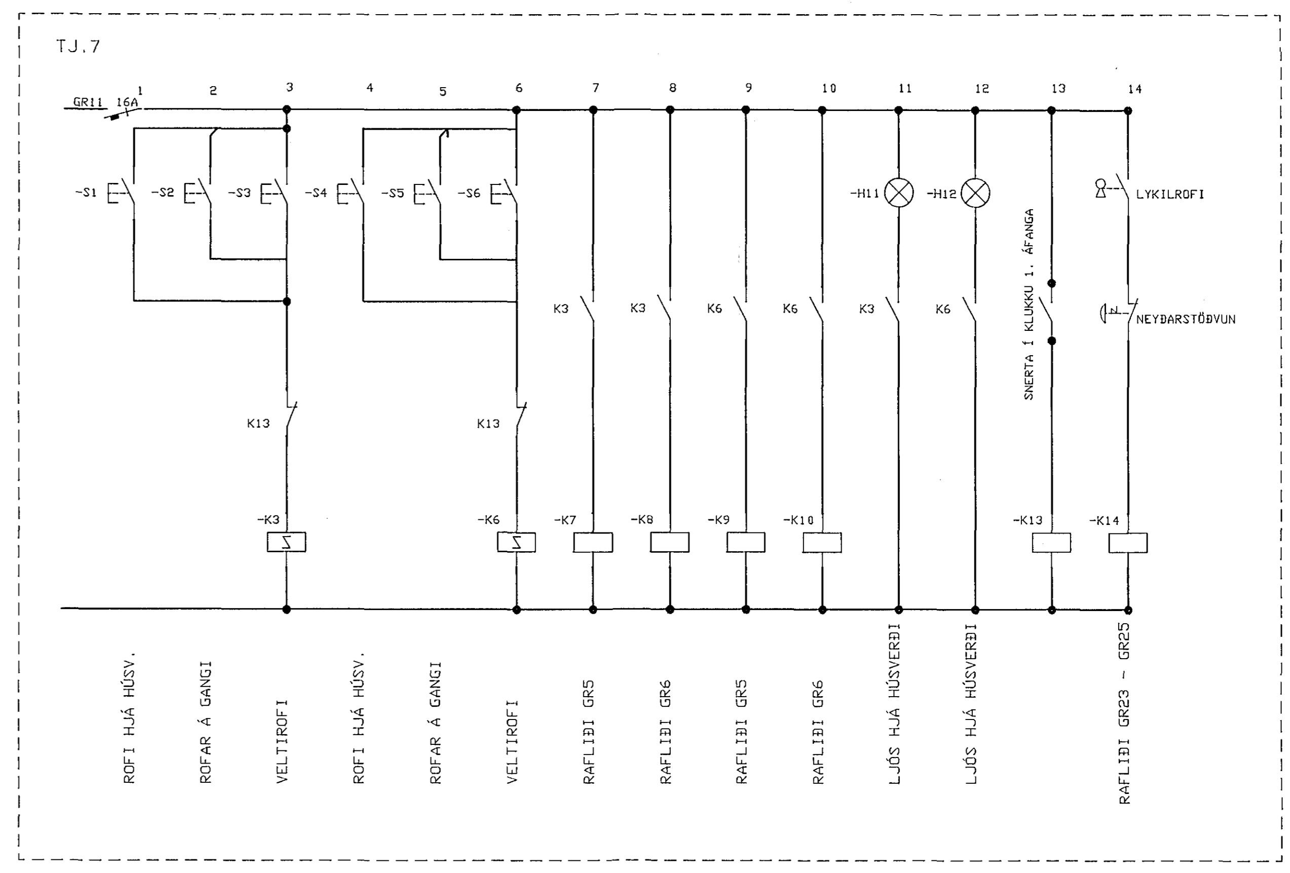
STYRING F. LJÓS Á GANGI 1.HÆÐ
