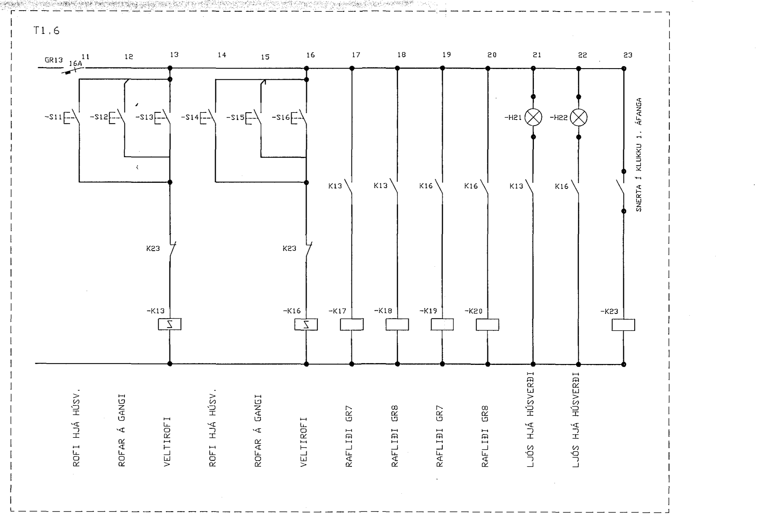
STYRING F. LJÓS Á GANGI 2.HÆÐ
