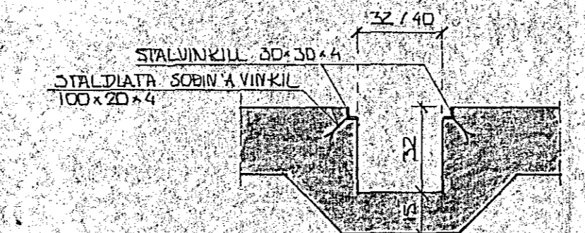
SNID B-B Mkv. 1:20
