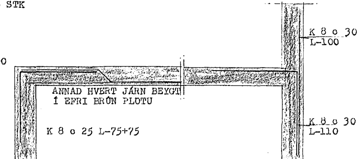
SNID - C 1:20
