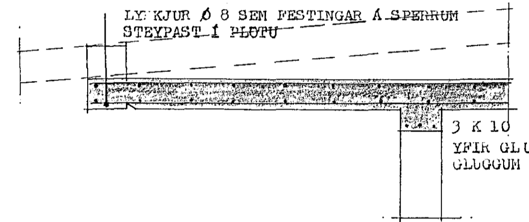
SNID - E 1:20
