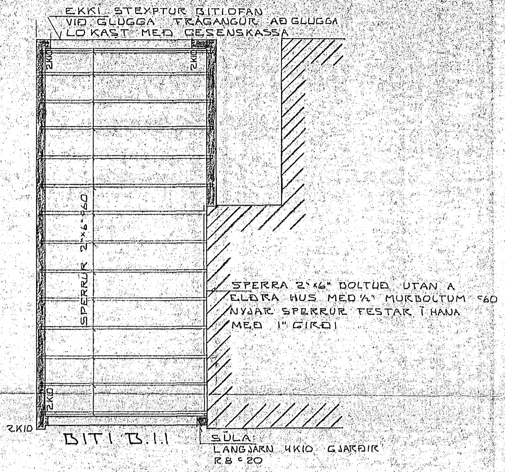
GRUNNMYND 1:50
