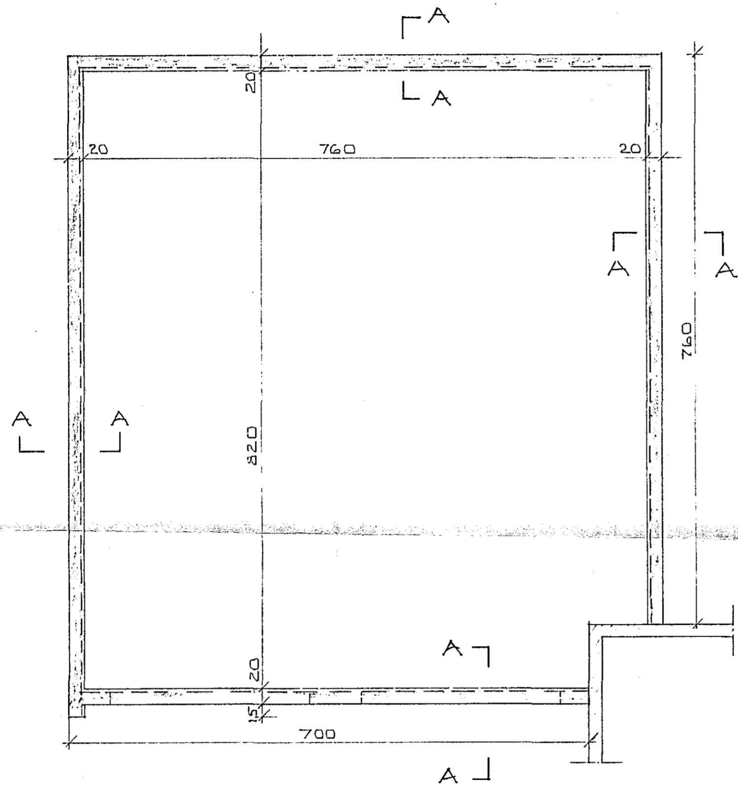
GRUNNMYND 1:50
