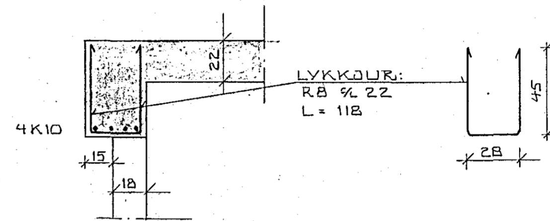
SNÍÐ B - B 1:20
