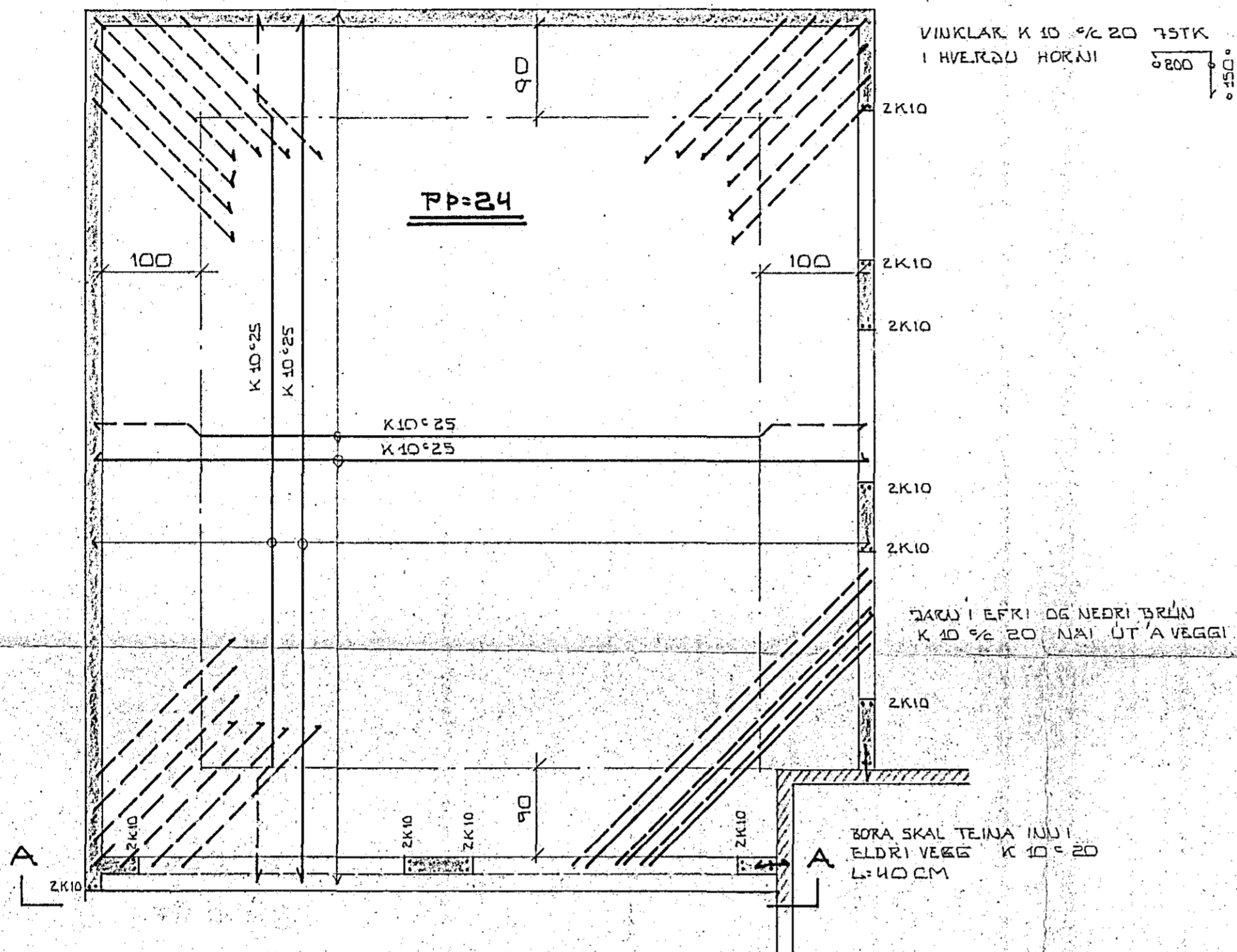
GRUNNMYND BÍLGEYMSLU 1:50
