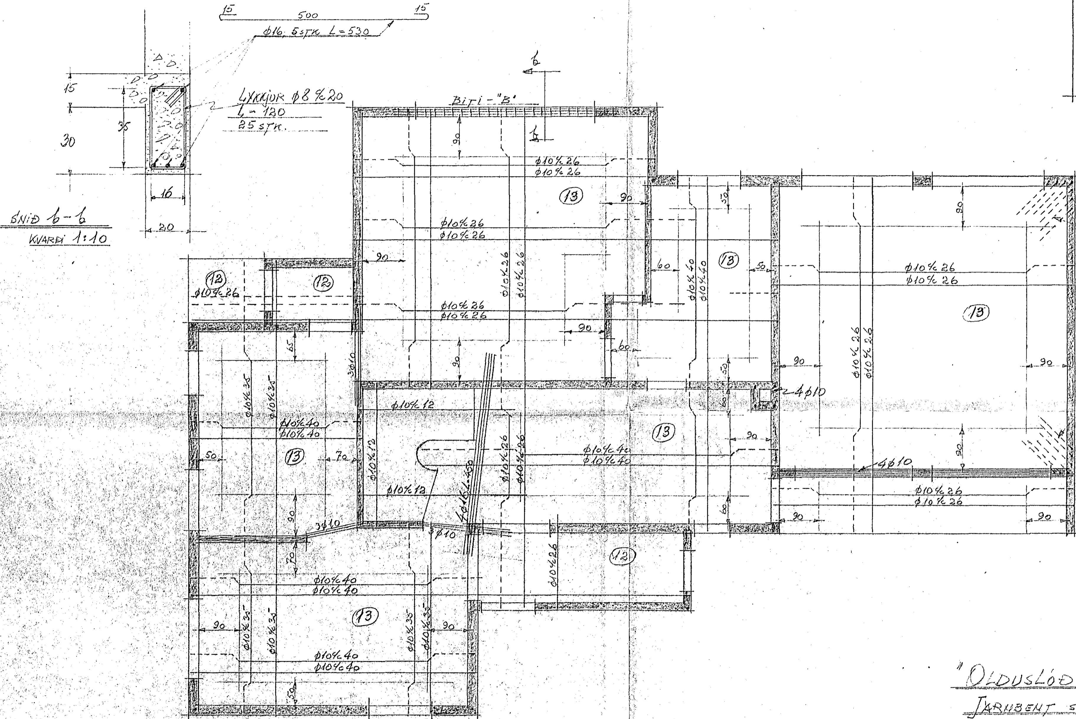
GRUNNMYND KVARNI 1:50
