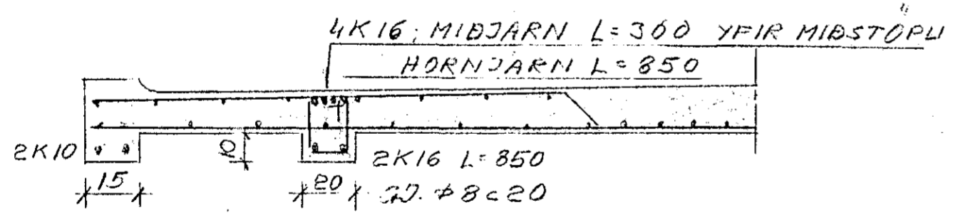
B-B 1:20
