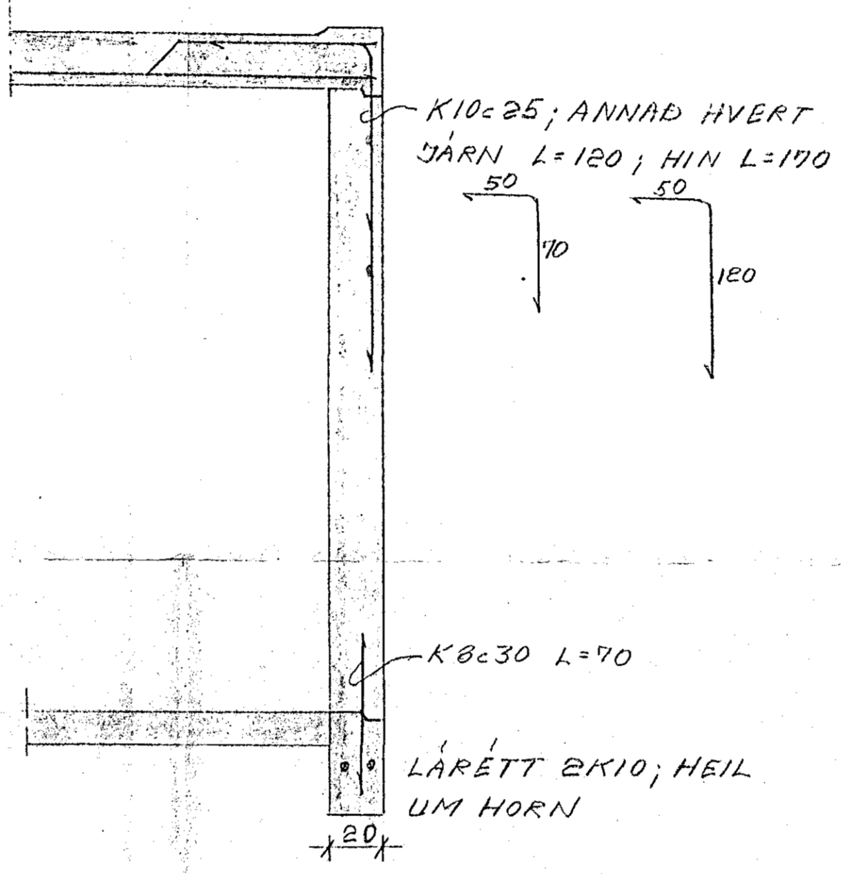
A-A 1:20
