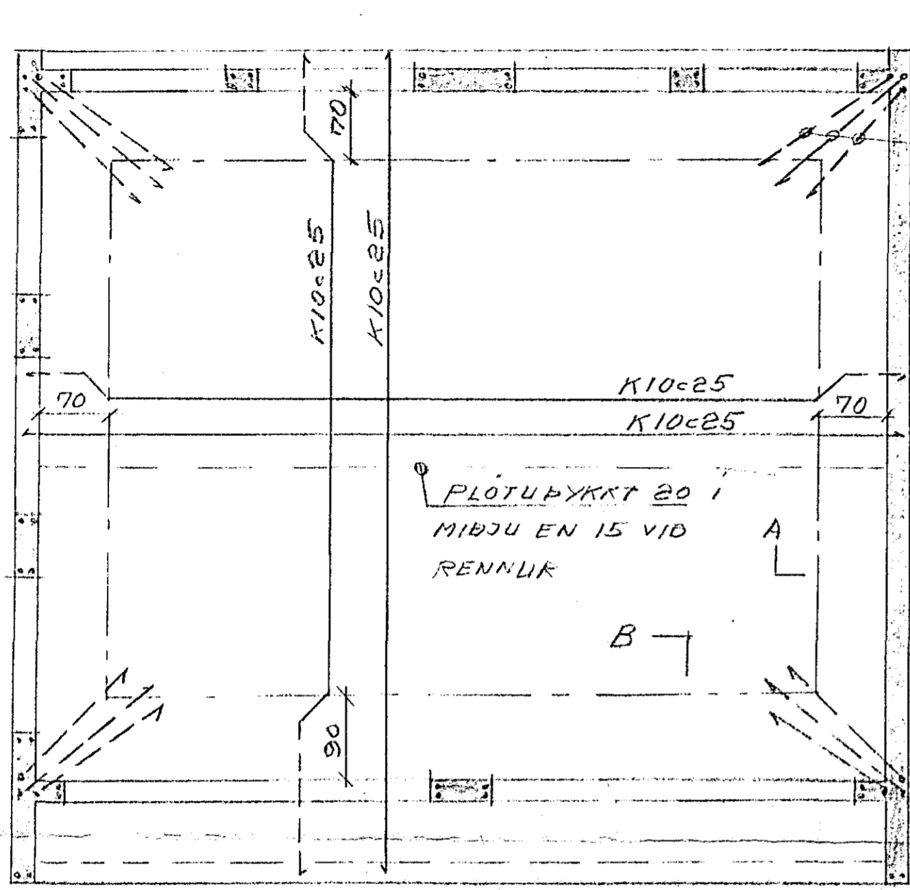
GRUNNMYND PAKPLOTU - 1:50 -
