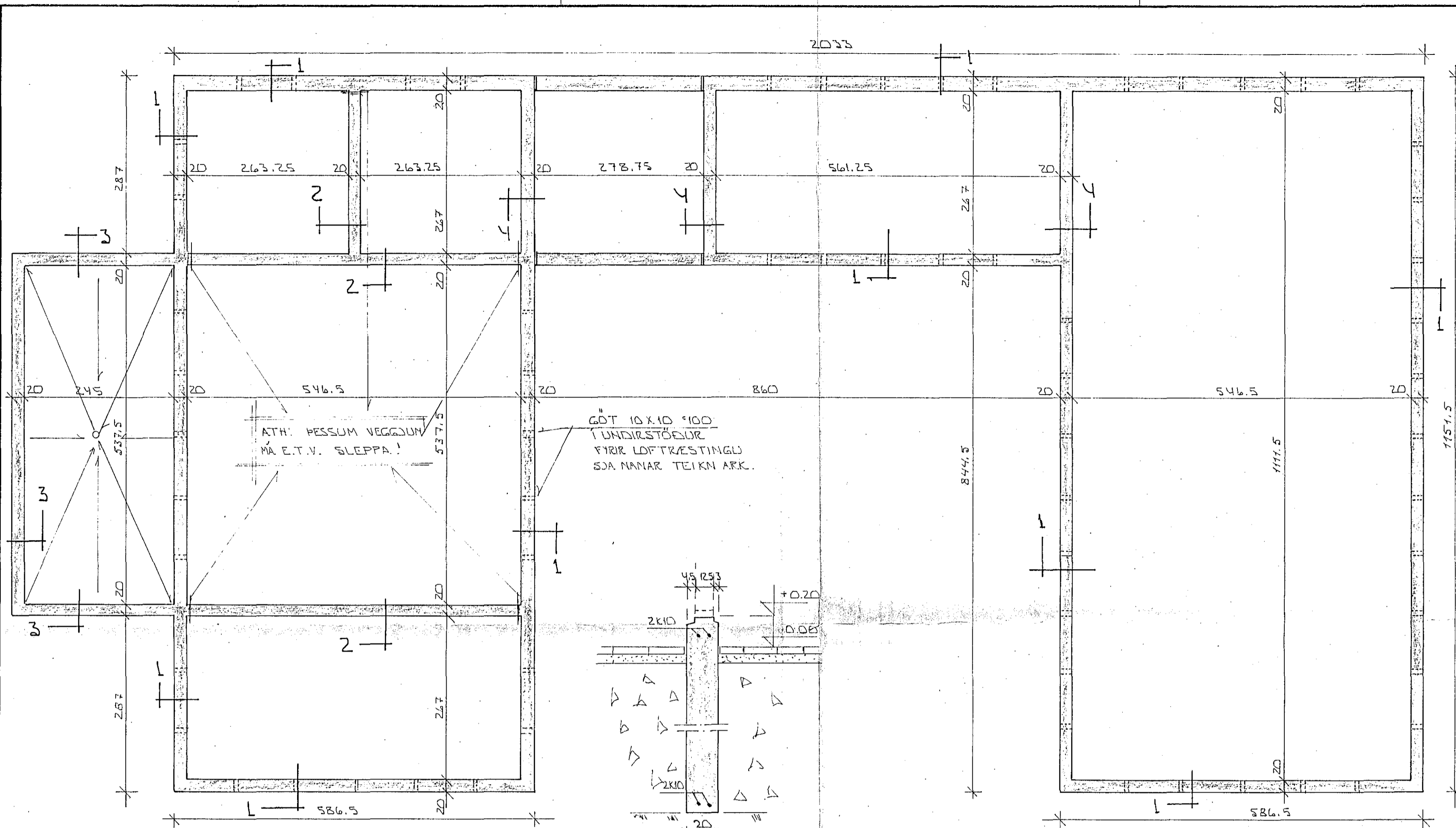
GRUNNMÝND • 1:50
