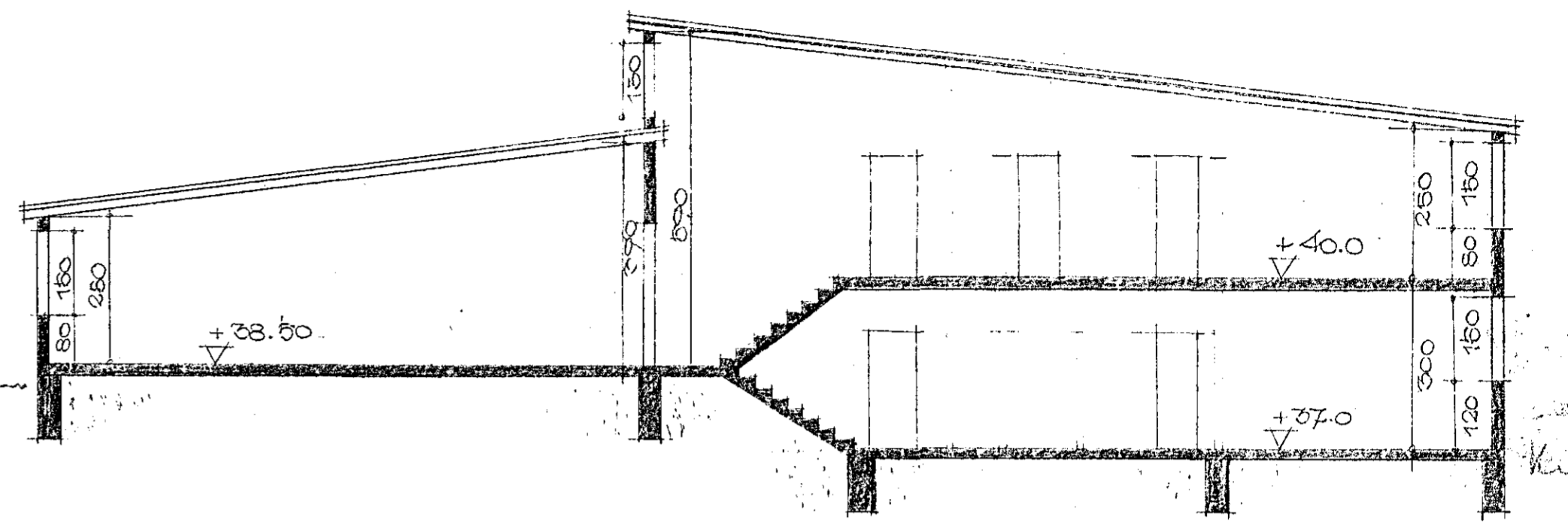
SNITT UM SKALA OG STIGAHÚS
