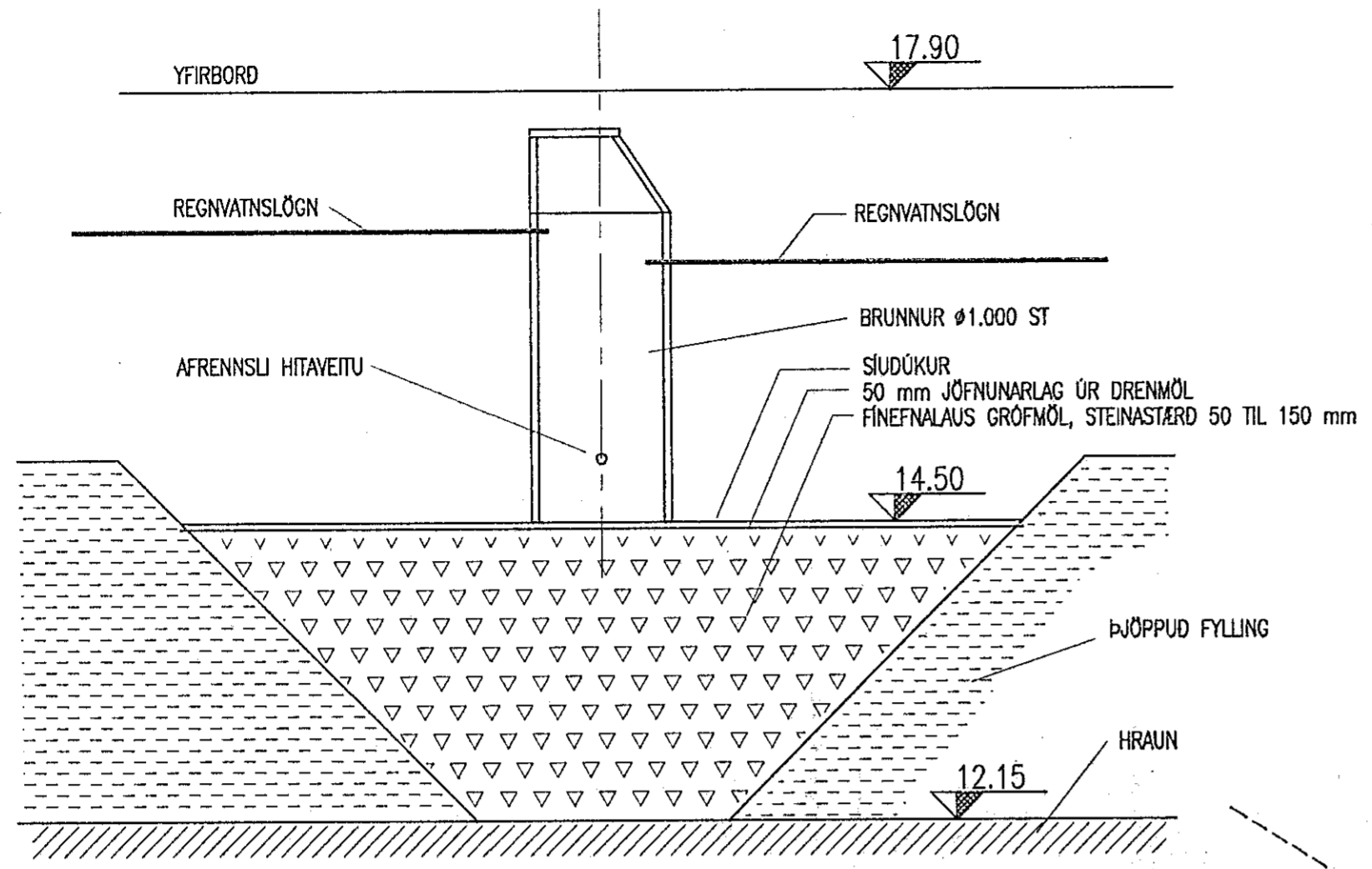
SNID Í SVELGBRUNN 1:50
