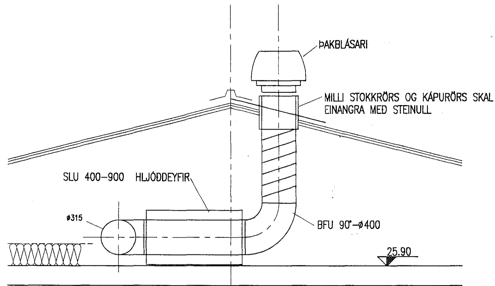
SNÍÐ Í RISHÆÐ OG ÚTSOGSKERFI 1:20
