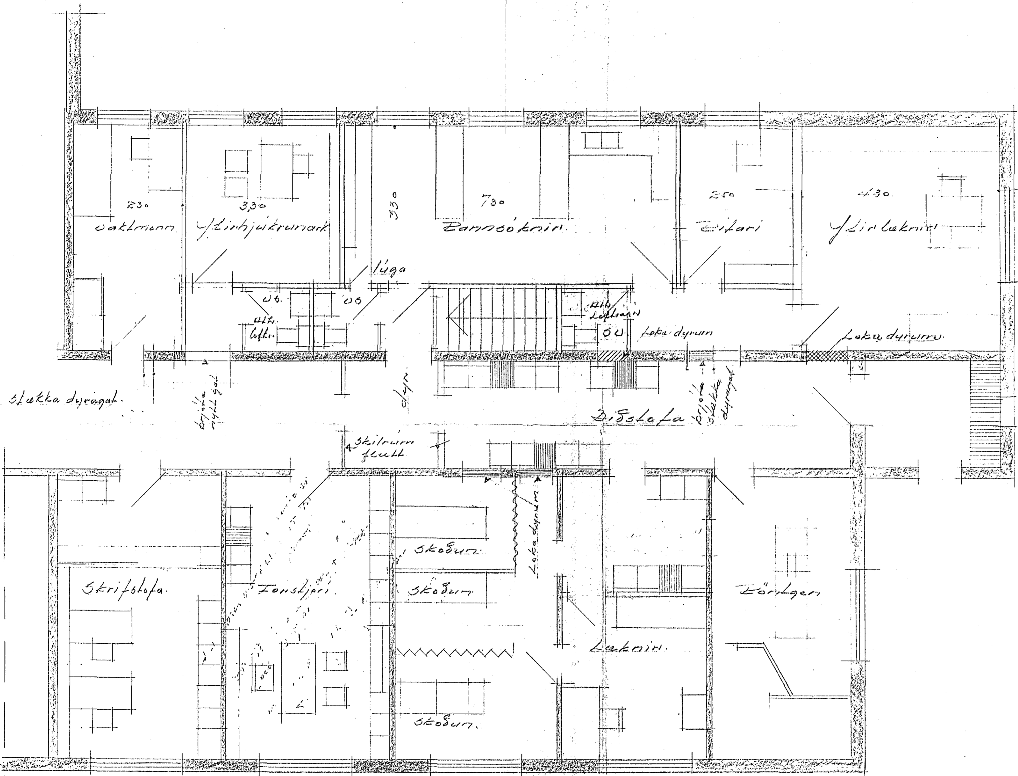
GRUNNMYND 1.4 AUSTURENDI 1:150.
