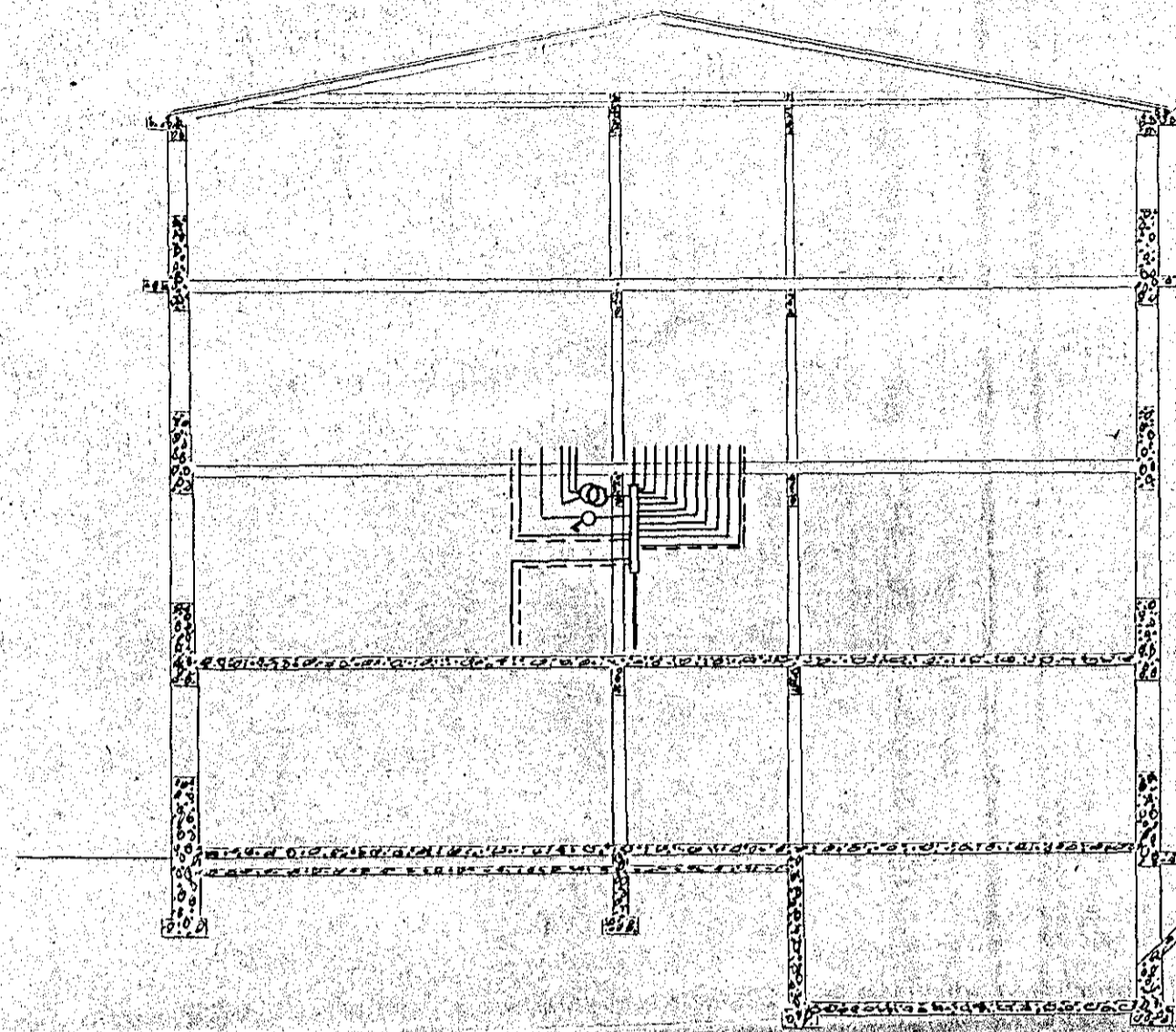
Þverskurður
