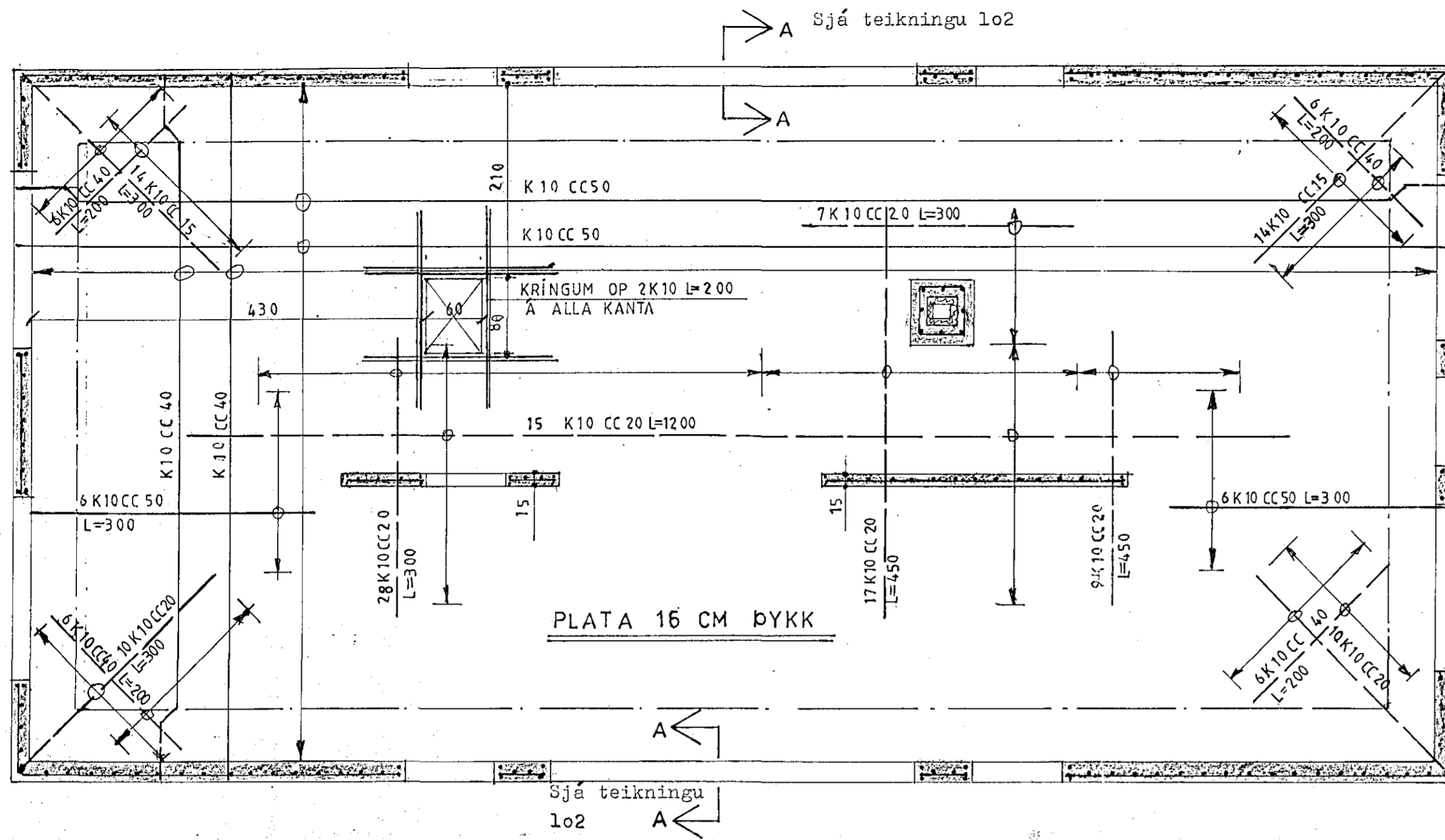
PLATA YFIR ÍBÚÐ M;1:50
