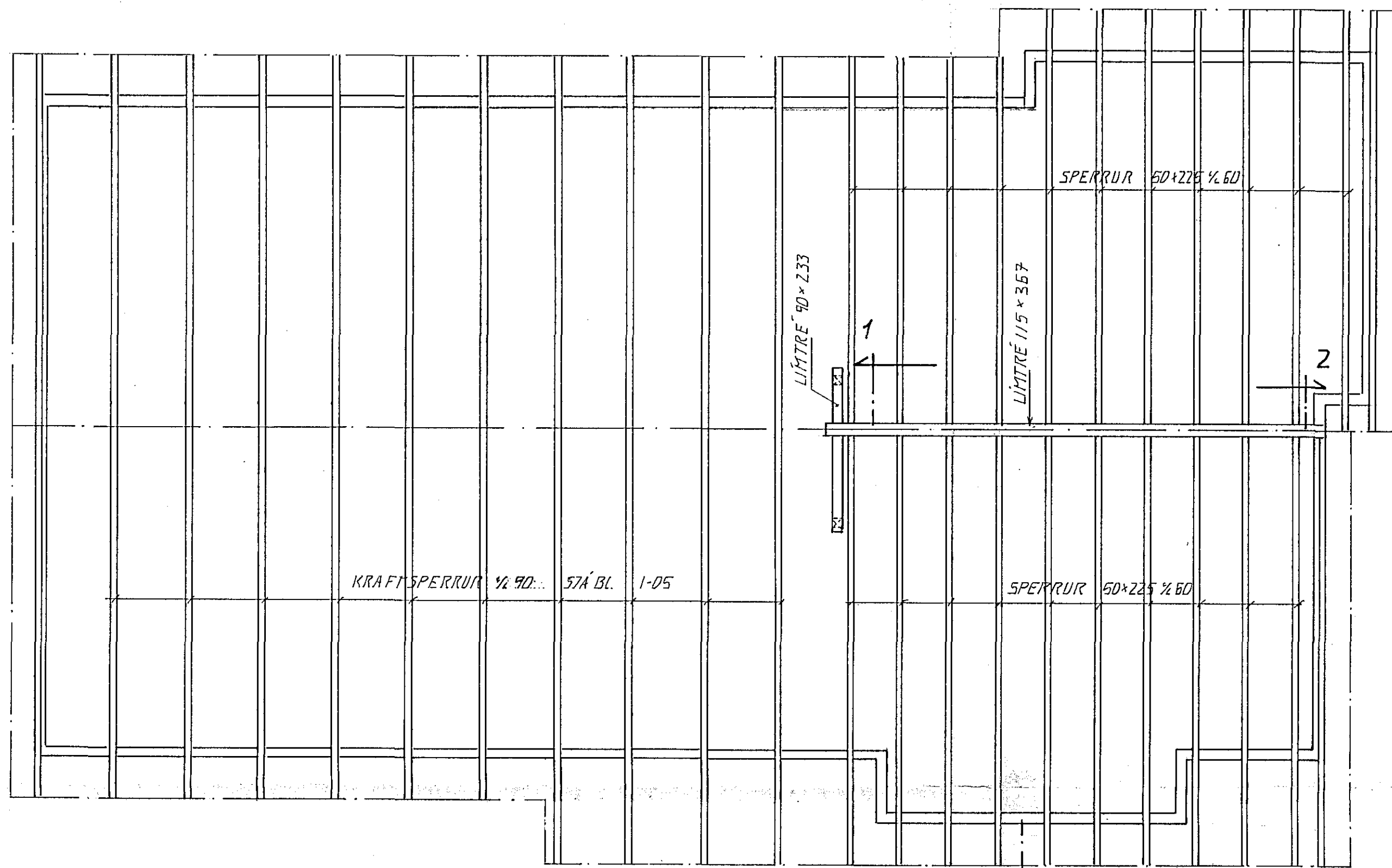
GRUNNMYND PAK. 1:50
