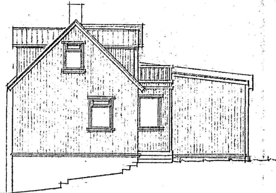
SUÐ-VESTUR 1:100
