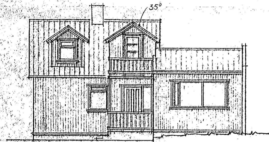
SUÐ-AUSTUR 1:100
