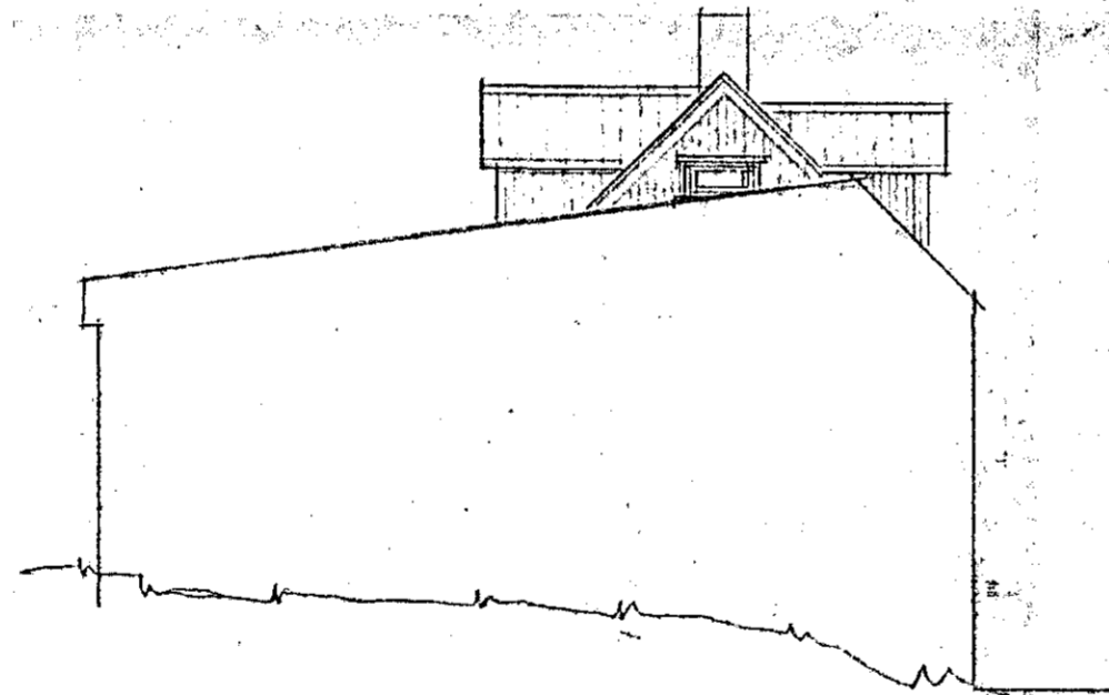
NÖRÐ-AUSTUR 1:100
