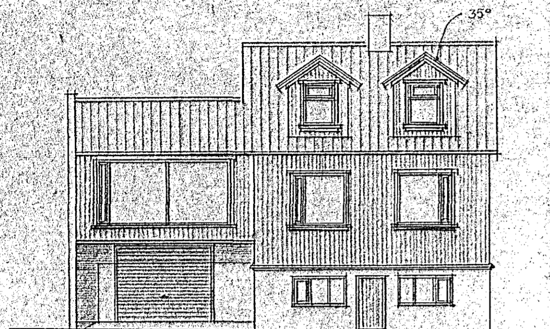
NORÐ-VESTUR 1:100
