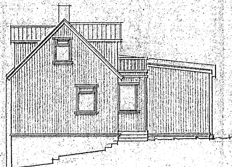
SUÐ-VESTUR 1:100
