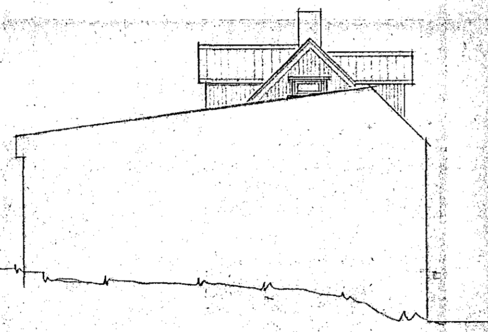
NORÐ-AUSTUR 1:100
