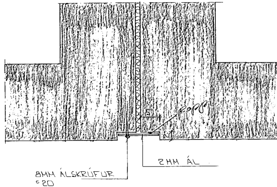
SÉRMYND A FRÁGANÐUR ÞENNSLUKILA x 1:5
