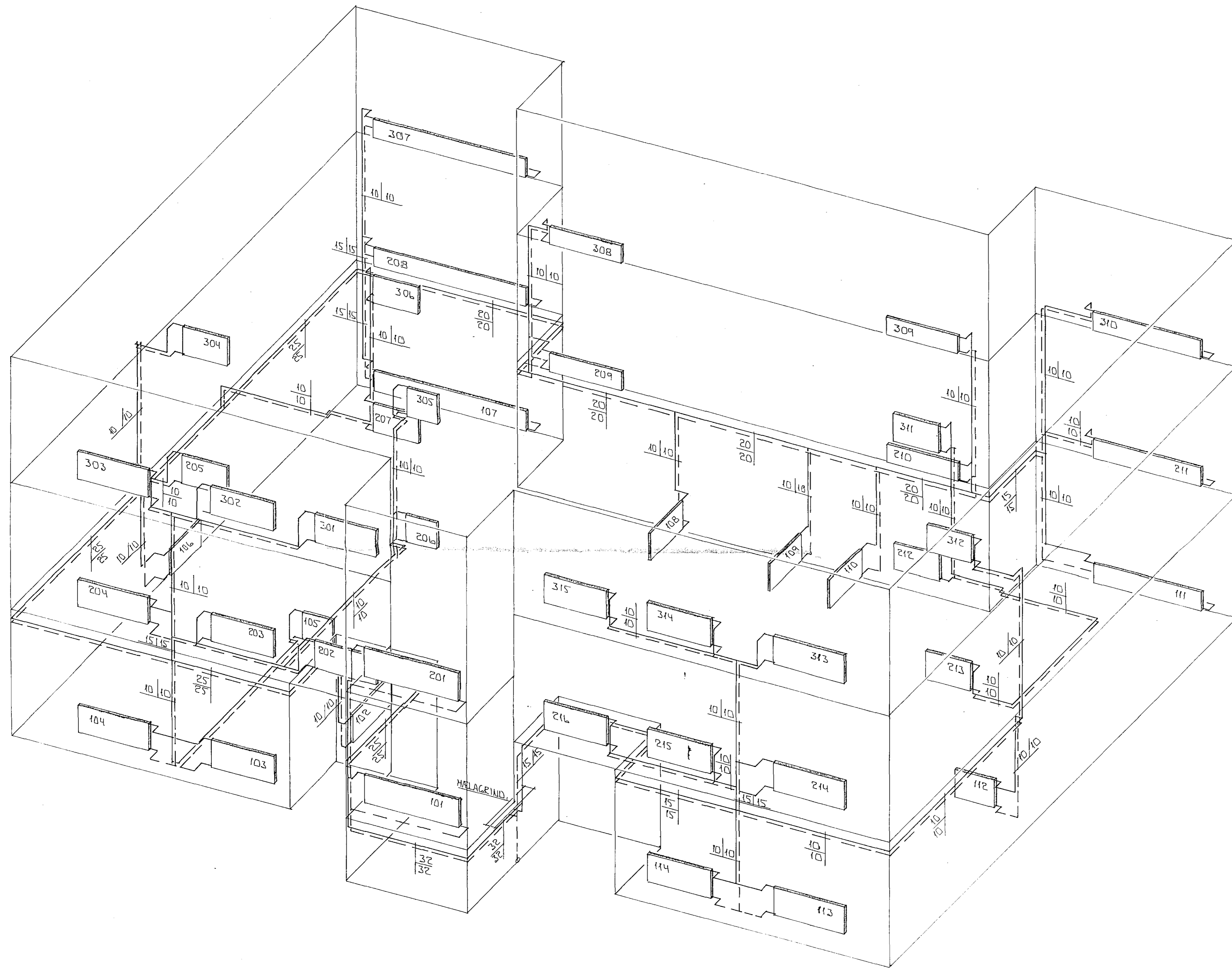
RÚMMYND HITALAGNA 1:50
