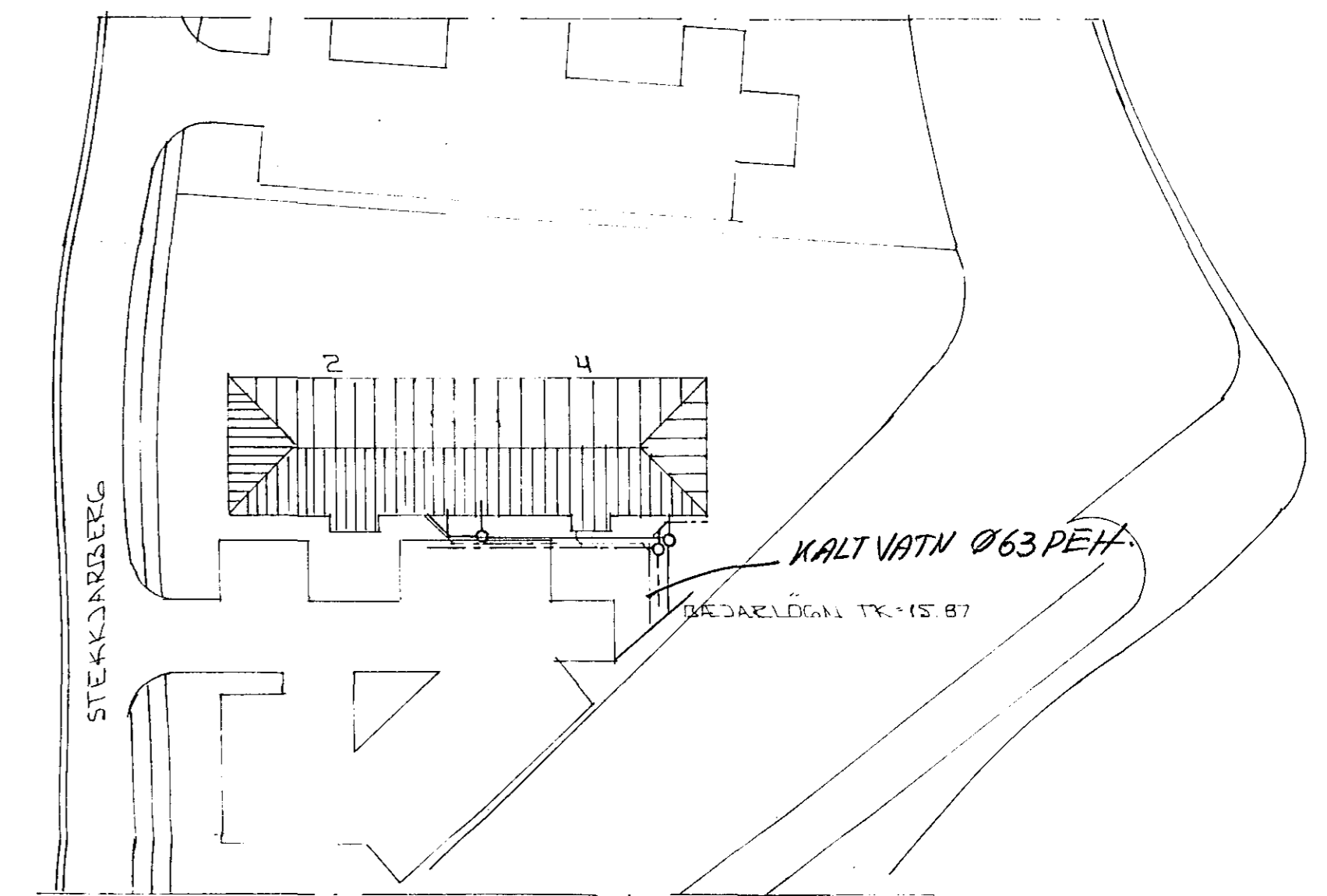
AFSTÖÐUMYND 1:500
