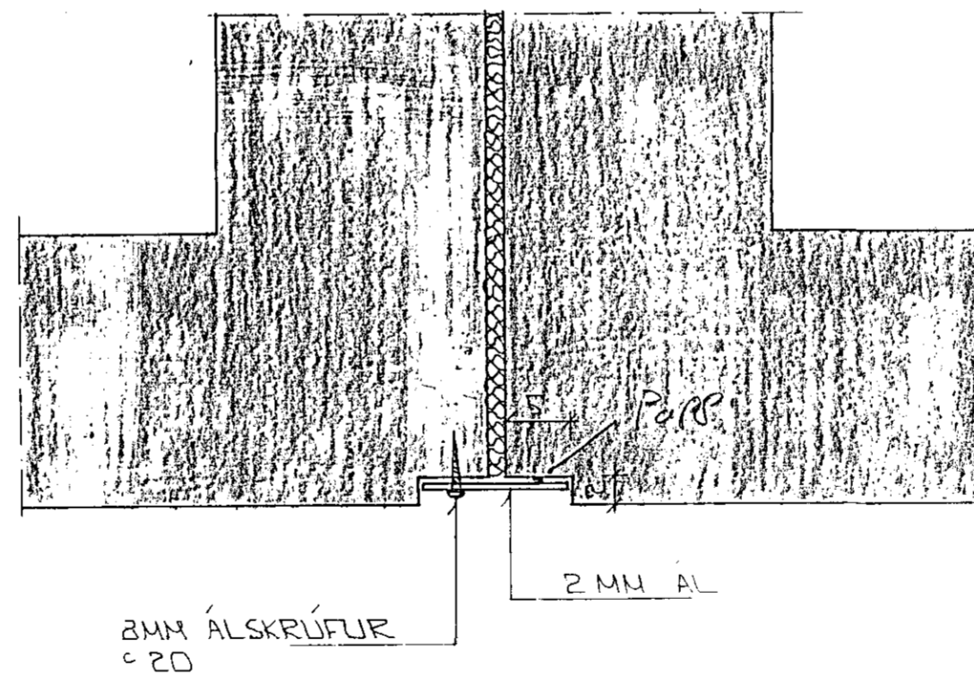
SÉRMYND A FRÁGANGUR PENNSLUSKILA x 1:5
