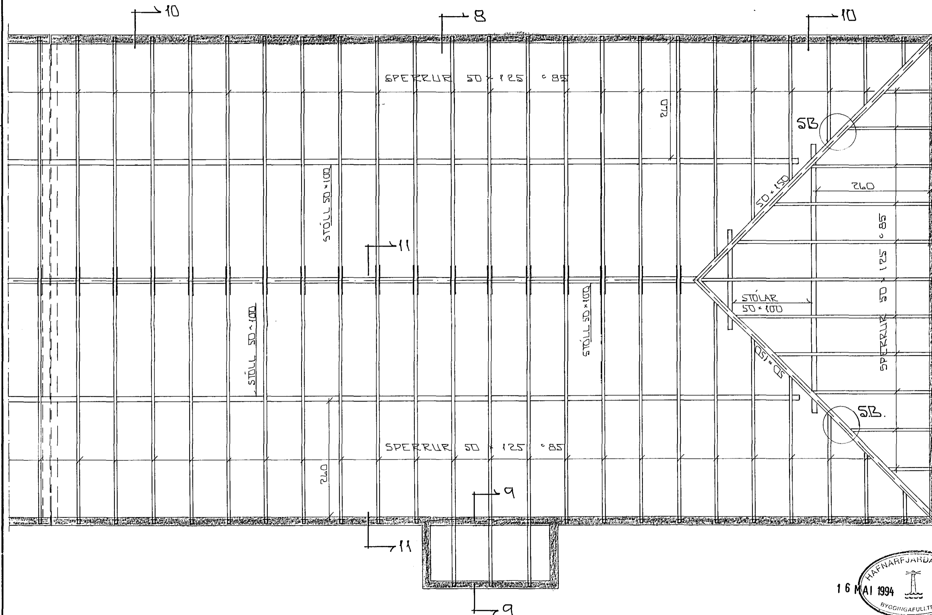
GRUNNMYND 1:50
