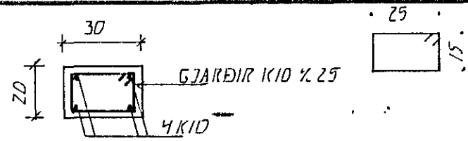
SÚLA S.1. 1:20
