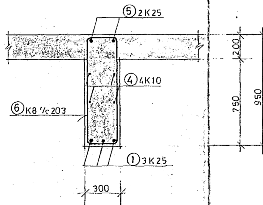
SNID B-B 1:20
