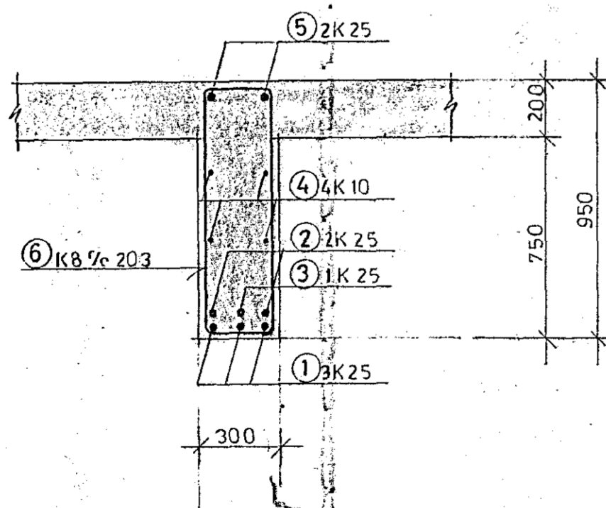
SNID A-A 1:20
