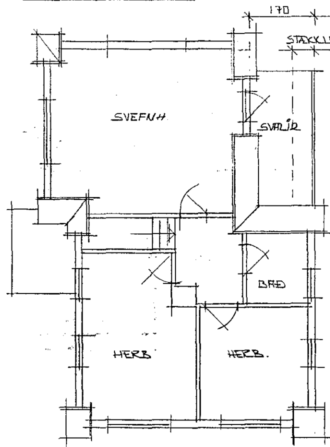
GRUNNMYND 1. HÆÐAR
