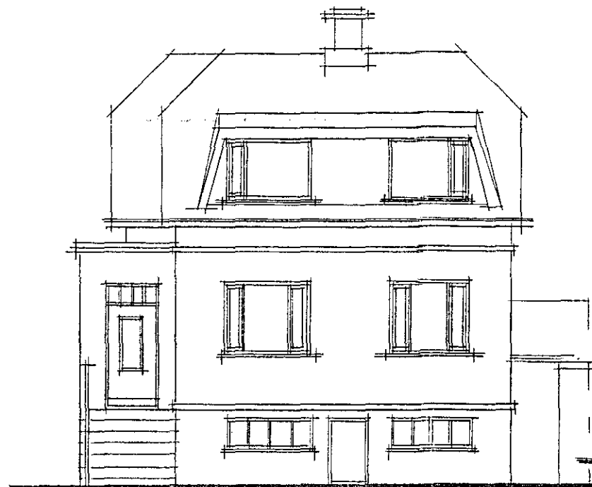
ÚTLIT NORÐUR
