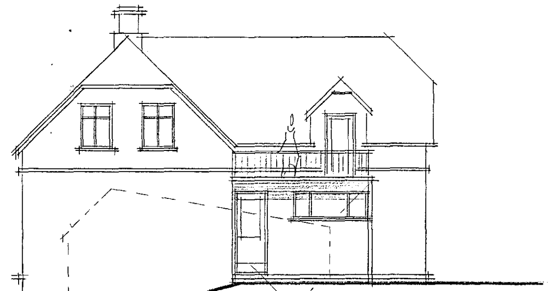
ÚTLIT AUSTUR
