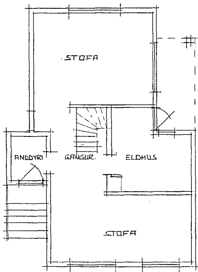
GRUNNMYND 1. HÆÐAR
