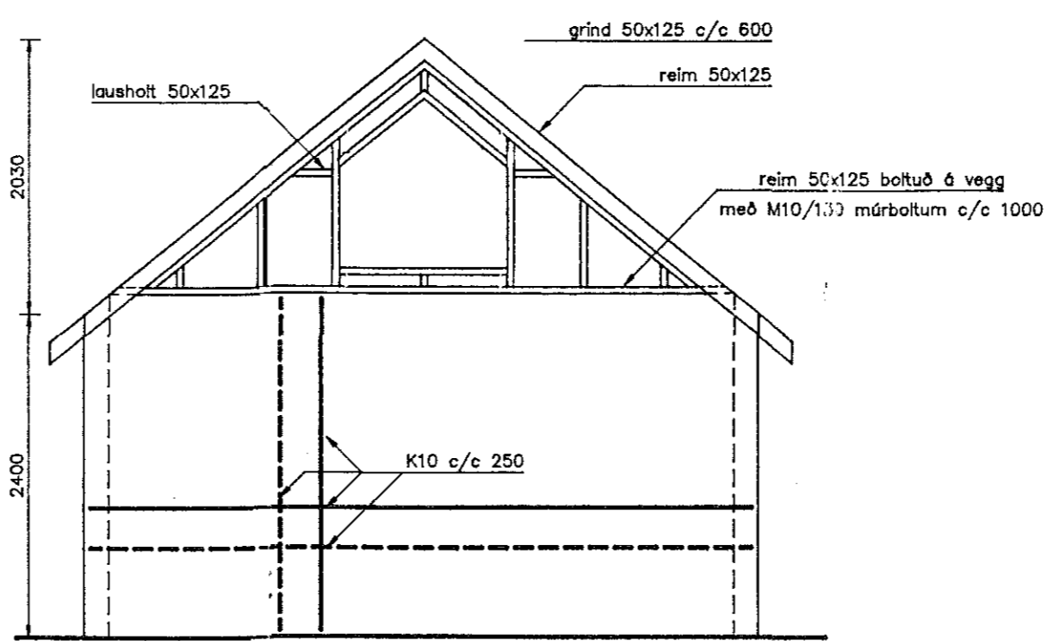
Suðurstafrn burðarvirki Mkv. 1: 50
