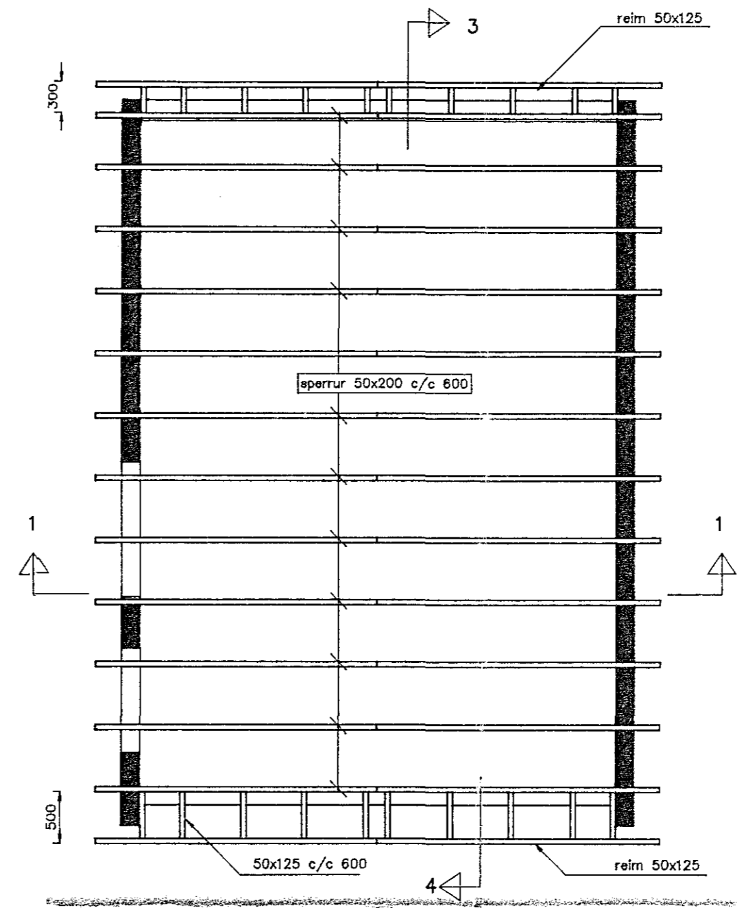
Grunnmynd þakviða Mkv. 1: 50
