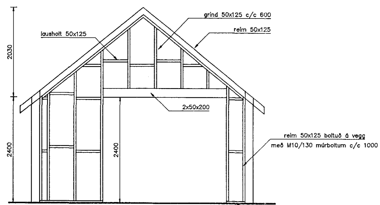
Timburgrind í stafni Mkv. 1: 50
