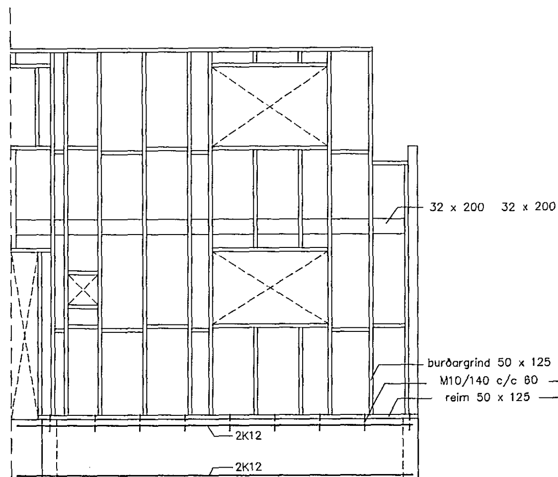
Burðarvirki norðurhliðar mkv. 1:50
