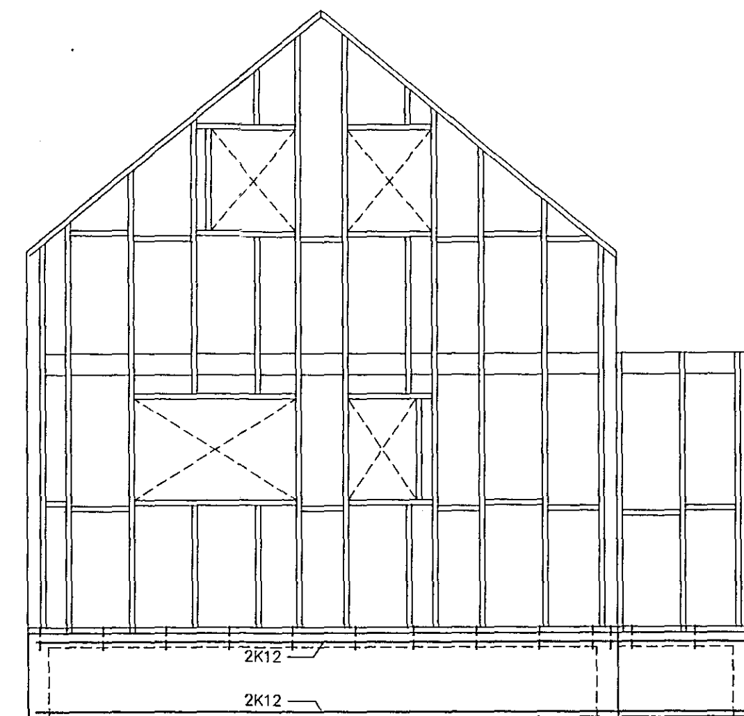
Burðarvirki vesturhliðar mkv. 1:50
