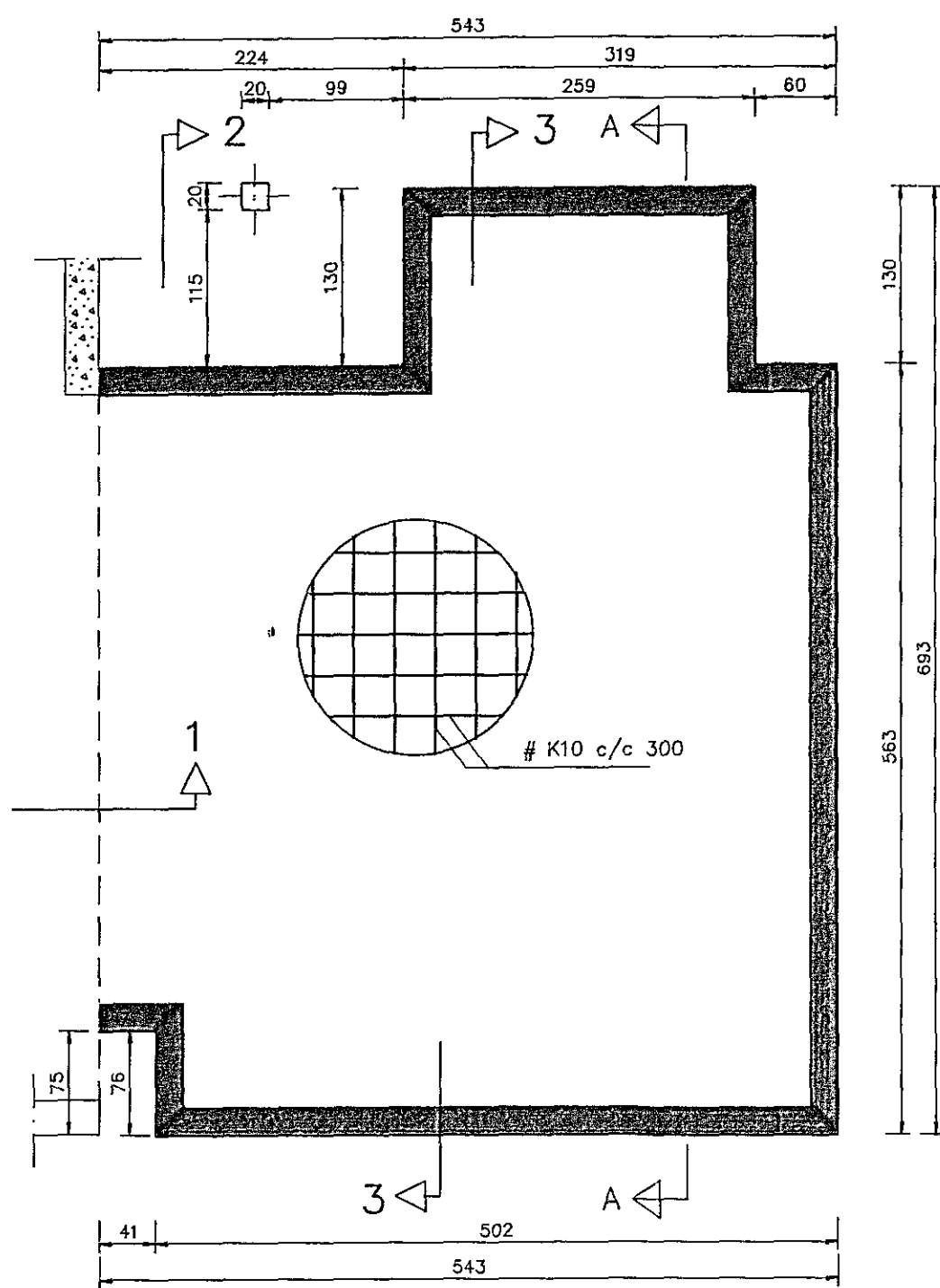
Grunnmynd sökklá mkv. 1:50
