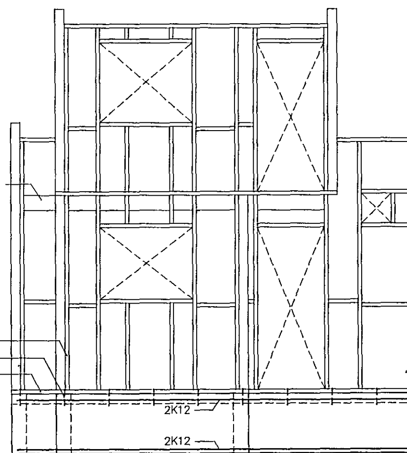
Burðarvirki suðurhliðar mkv. 1:50
