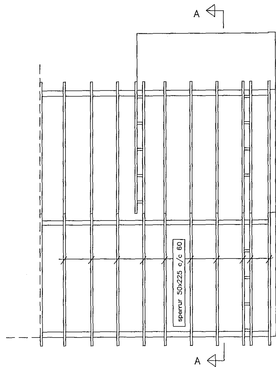
Grunnmynd þakviða mkv. 1:50
